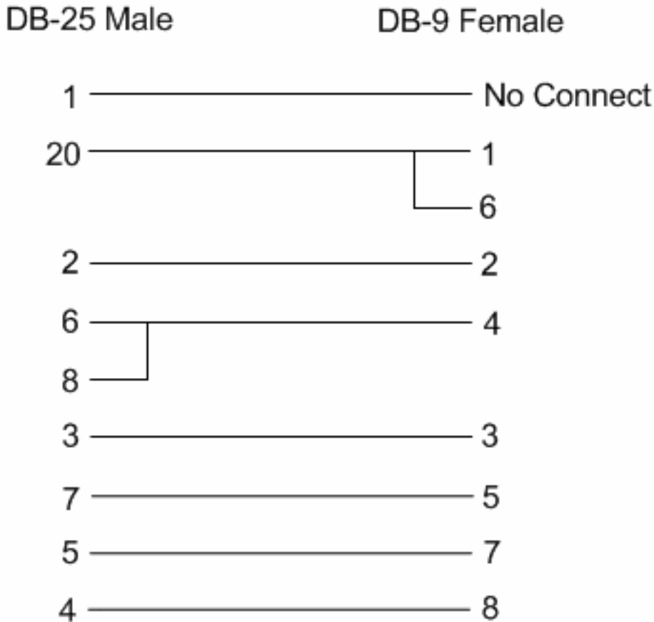
图1 – CRT电缆Pin缩小
