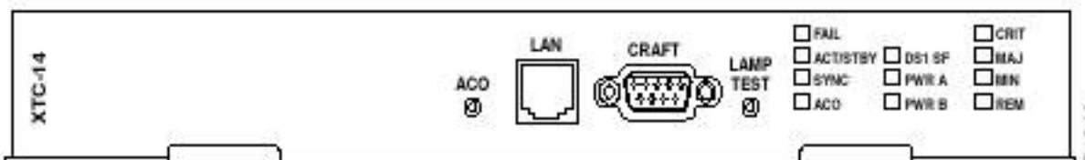
图 9. XTC-14 卡
