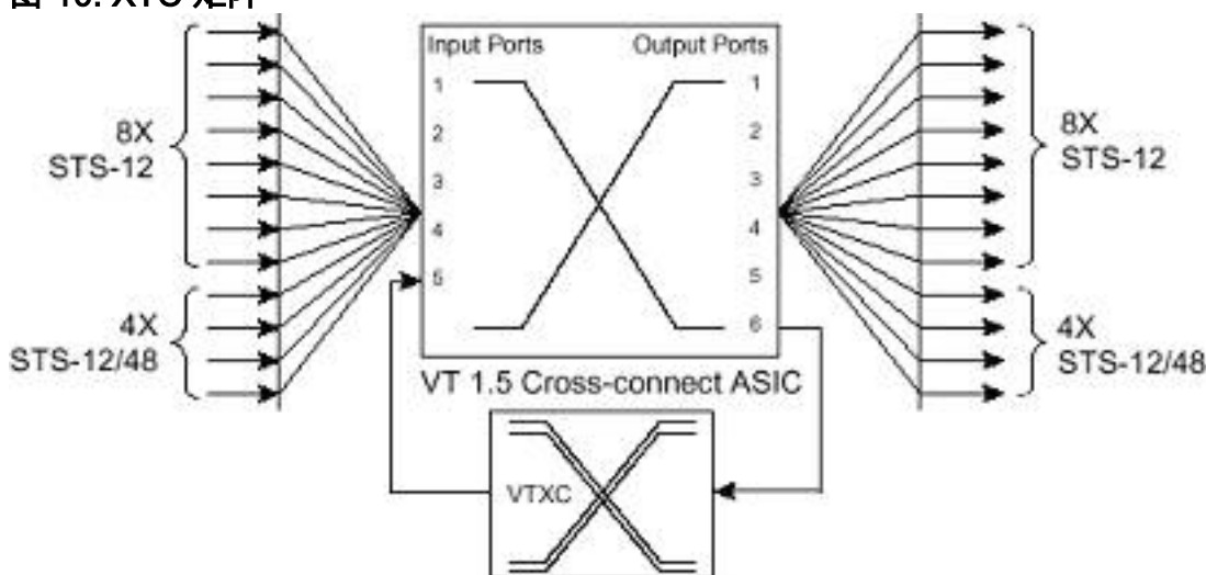
图 10. XTC 矩阵
