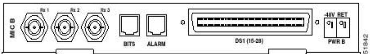
图 5. MIC 28-3-B 卡
