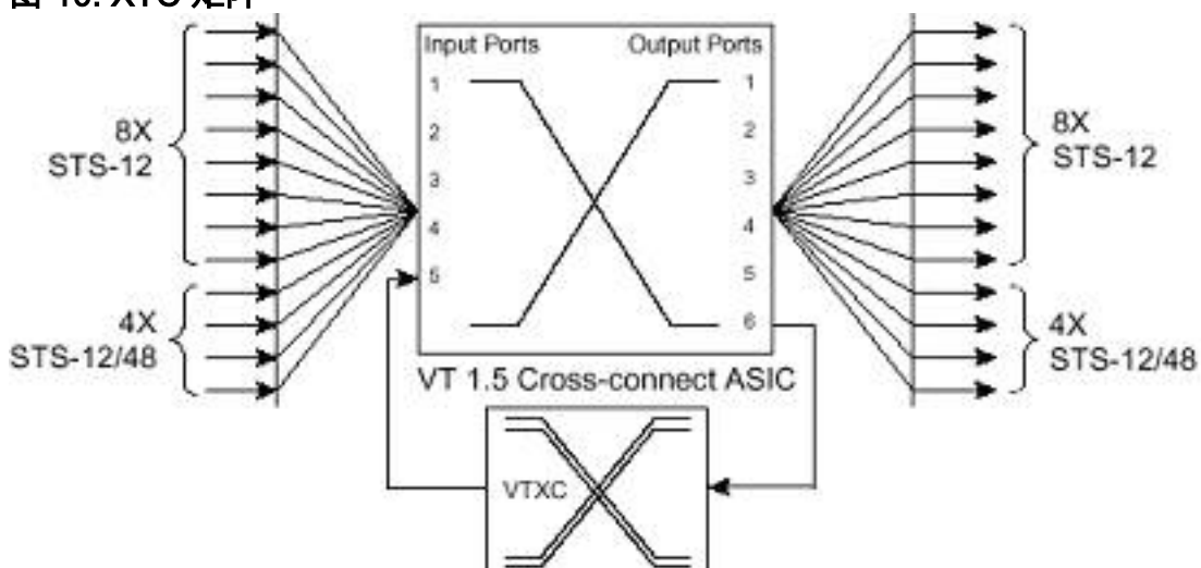
图 10. XTC 矩阵
