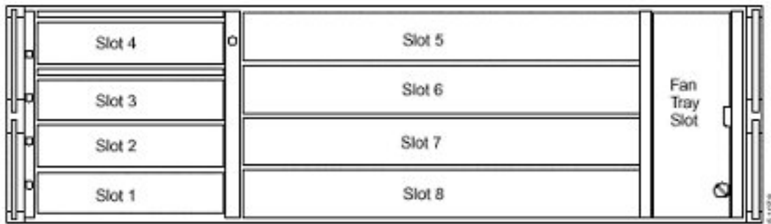
图 3. ONS 15327 机箱插槽编号
