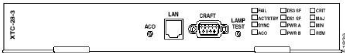
图 8. XTC-28-3 卡
