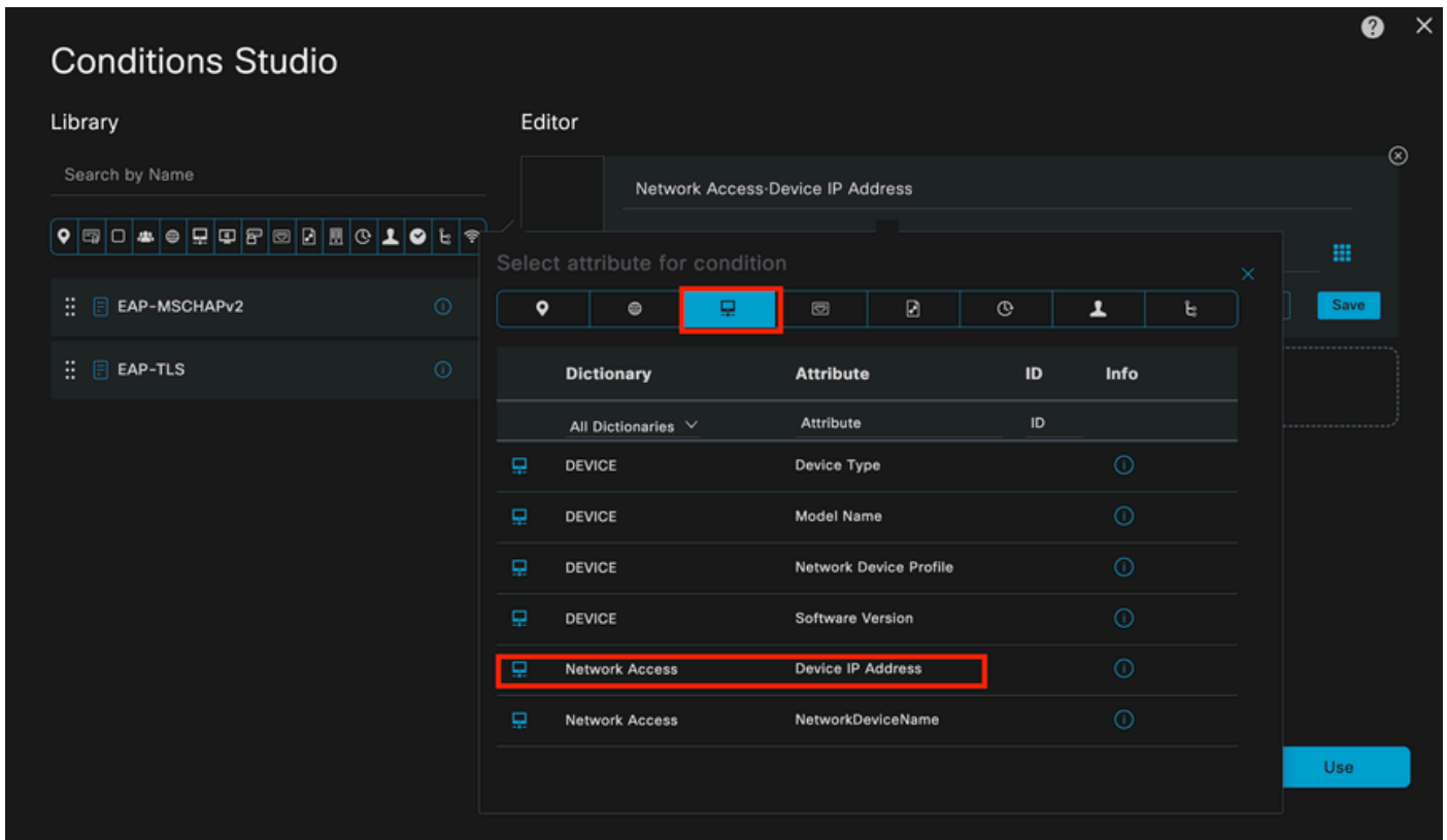
身份验证策略的Condition studio
