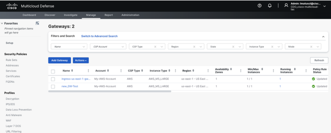
图 1.网关列表。
