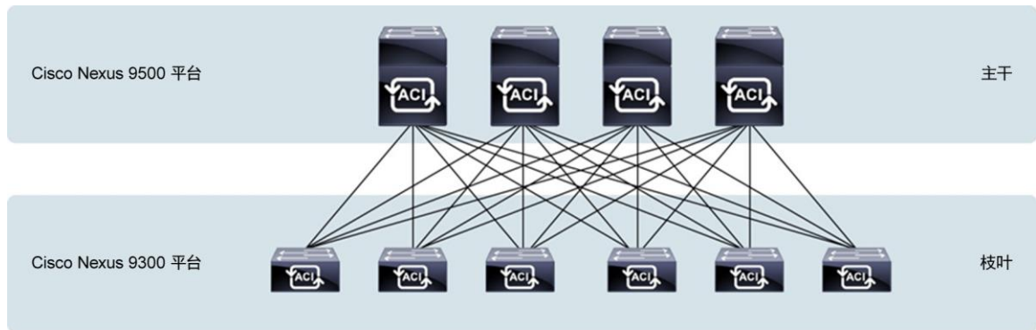
图 2. 枝叶和主干架构中的 Cisco Nexus 9500 平台
