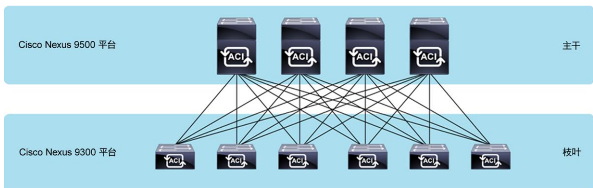
图 5. 枝叶和主干架构中的 Cisco Nexus 9500 平台
