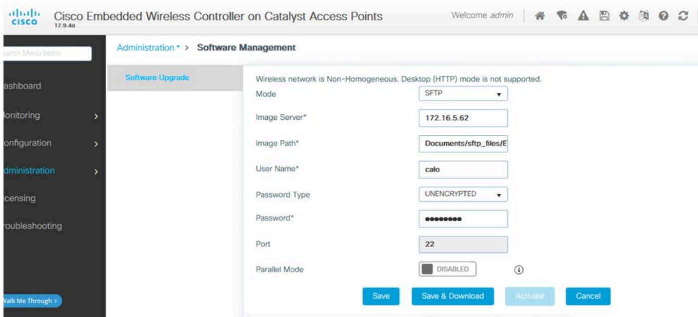
Configuração do SFTP na GUI
