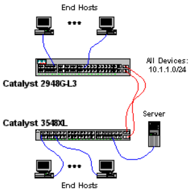
Figura 1: Diagrama da rede do exemplo 1
