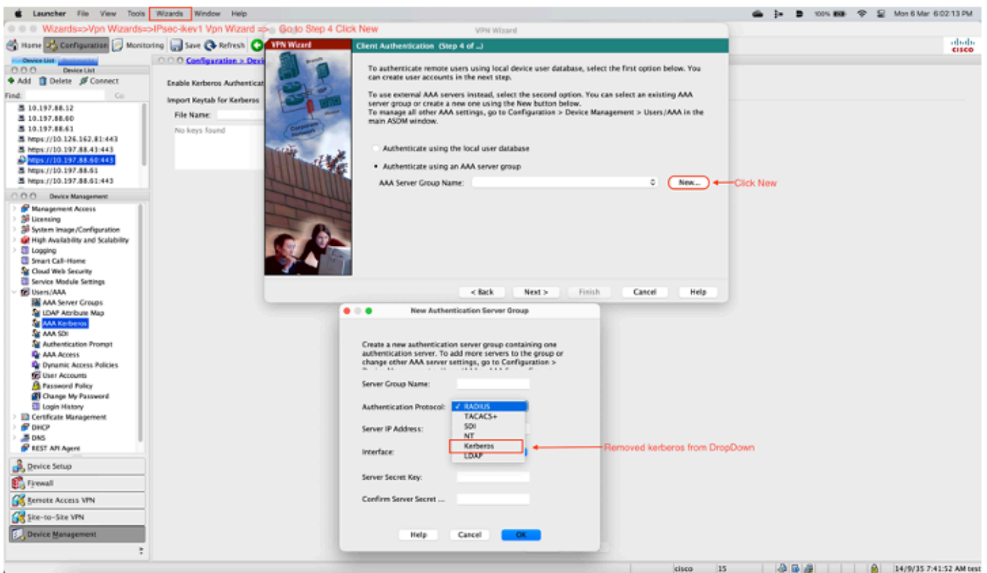
ASDM: Kerberos-protocol in nieuwe AAA-servergroep
