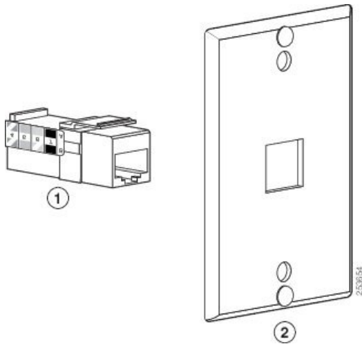
그림 21: Leviton 벽면 장착 플레이트
