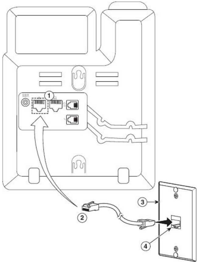
그림 23: 벽면 장착 책의 RJ45 커넥터
