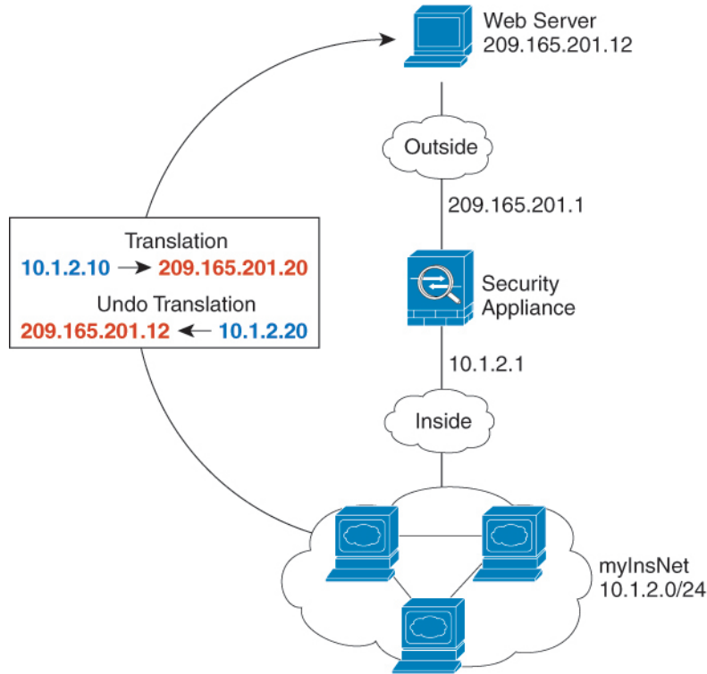
그림 16: 내부용 동적 NAT, 외부 웹 서버용 고정 NAT
