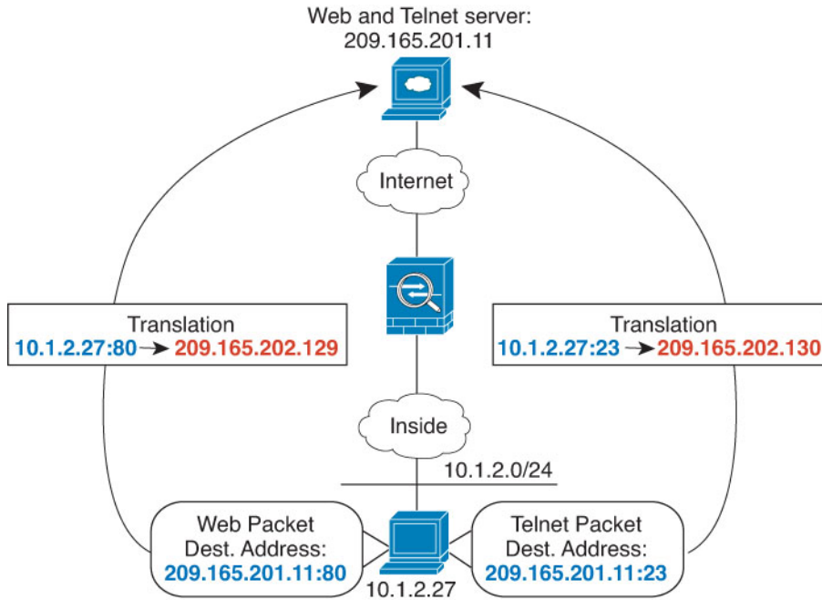
그림 20: 서로 다른 대상 포트를 사용하는 수동 NAT
