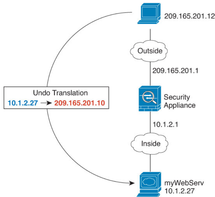
그림 15: 내부 웹 서버에 대한 고정 NAT
