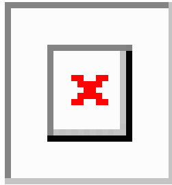
그림 8: 고정 NAT
