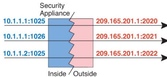
그림 7: 동적 PAT
