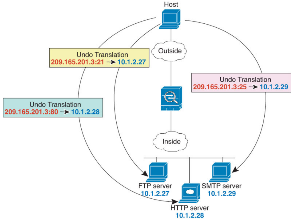
그림 18: 포트 변환 고정 NAT
