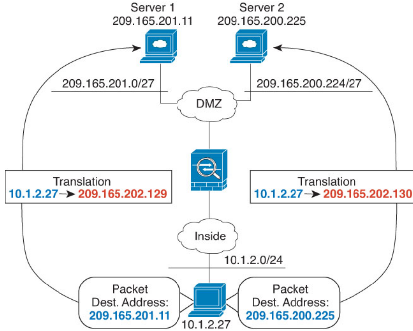
그림 19: 서로 다른 대상 주소를 사용하는 수동 NAT
