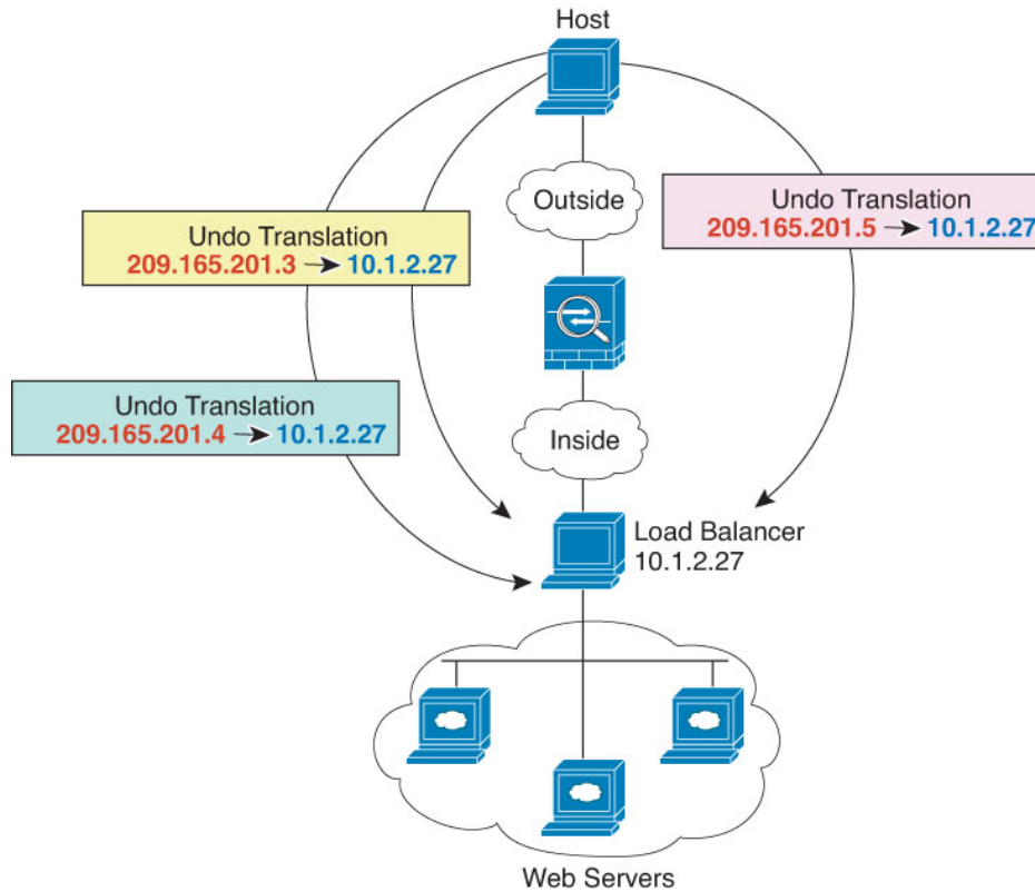
그림 17: 내부 로드 밸런서용 일대다 고정 NAT
