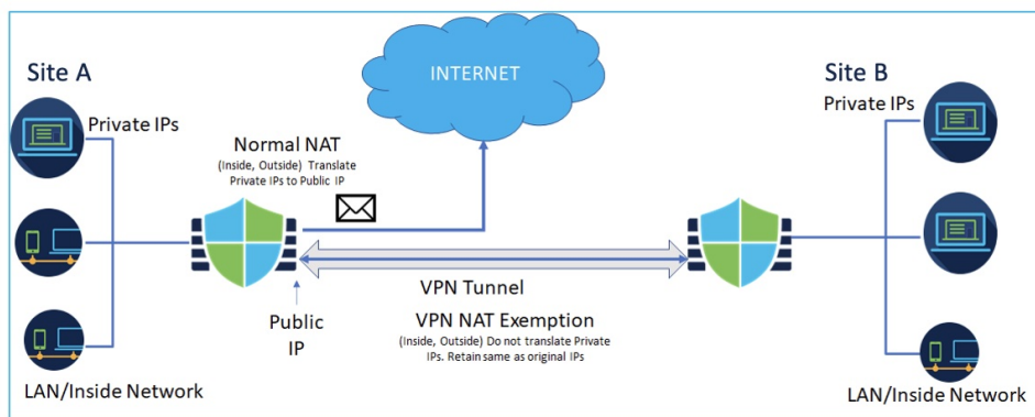
그림 4: NAT 제외 사이트 간 VPN 토폴로지
