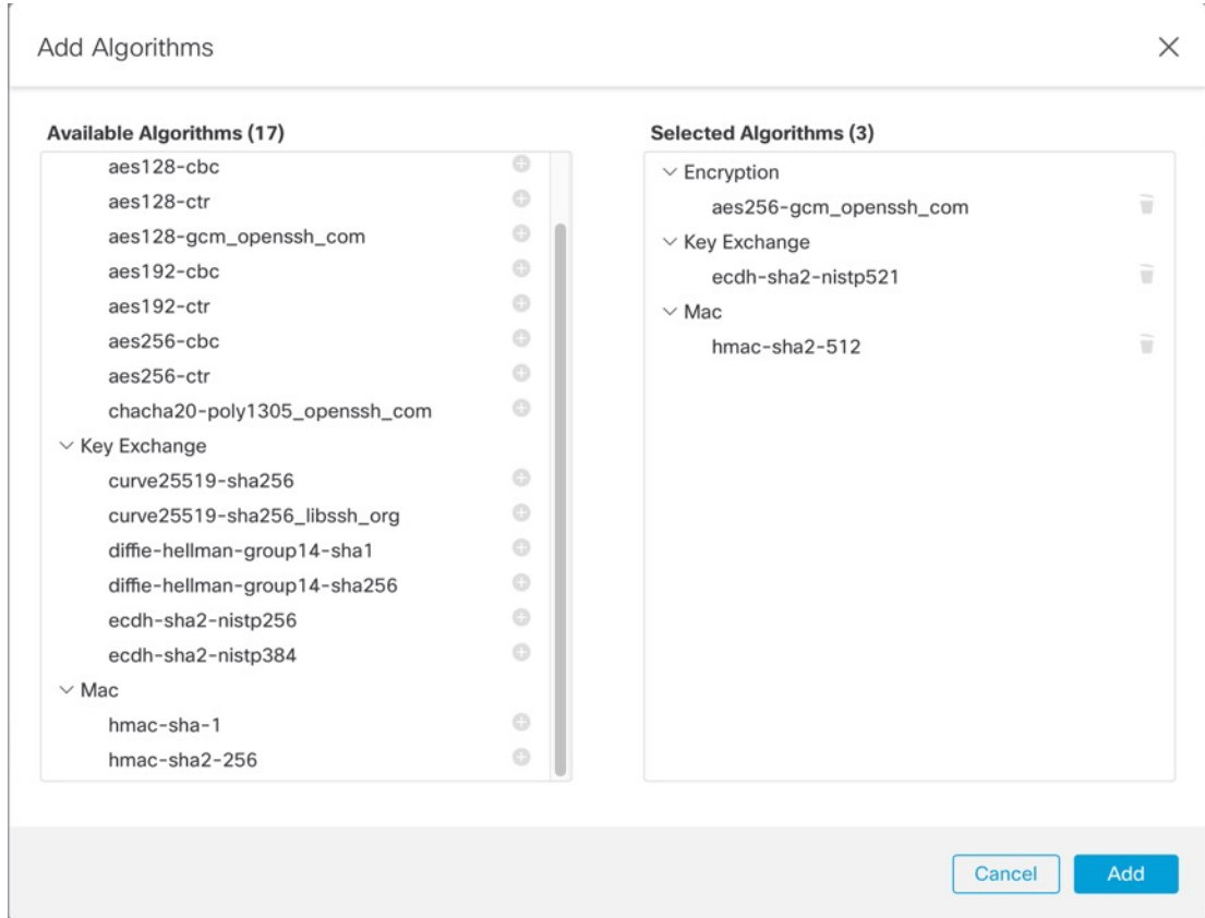
그림 47: □알고리즘추가
