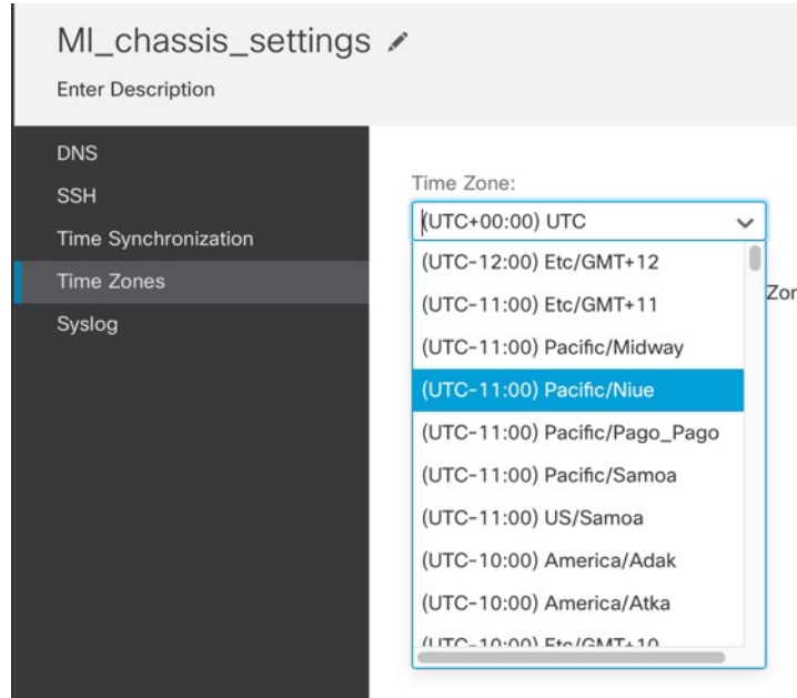
그림 57: 표준 시간대
