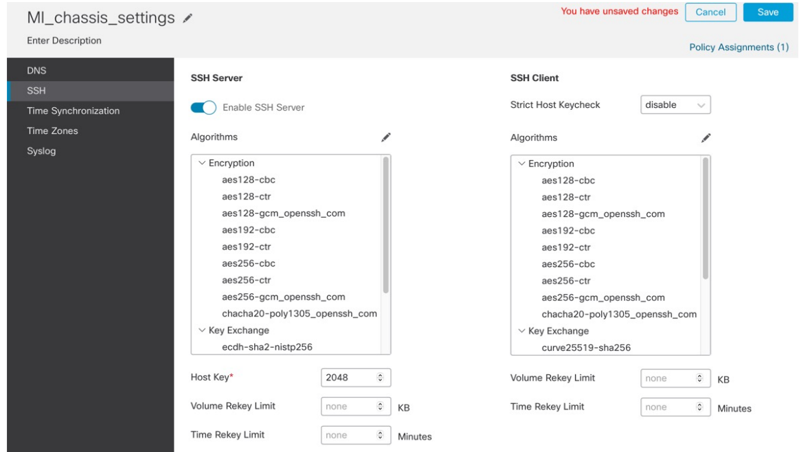
그림 48: SSH
