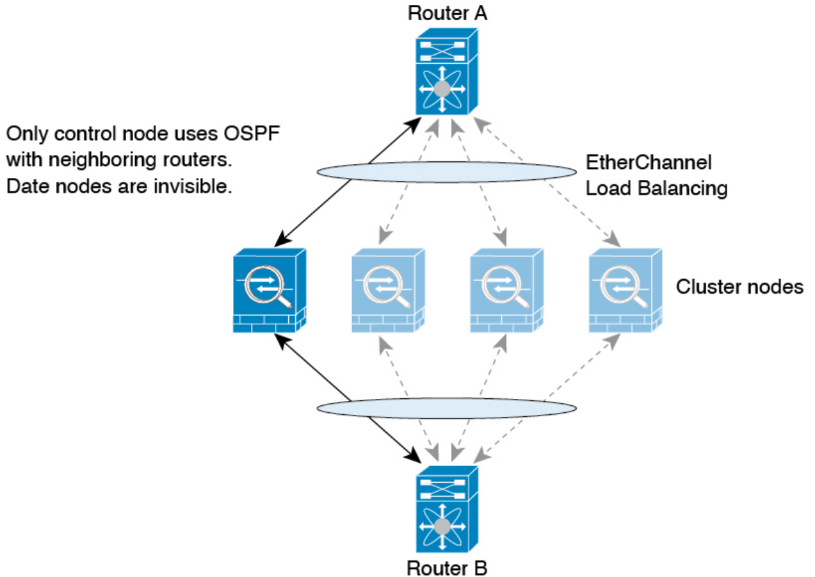
그림 33: Spanned EtherChannel 모드의 동적 라우팅
