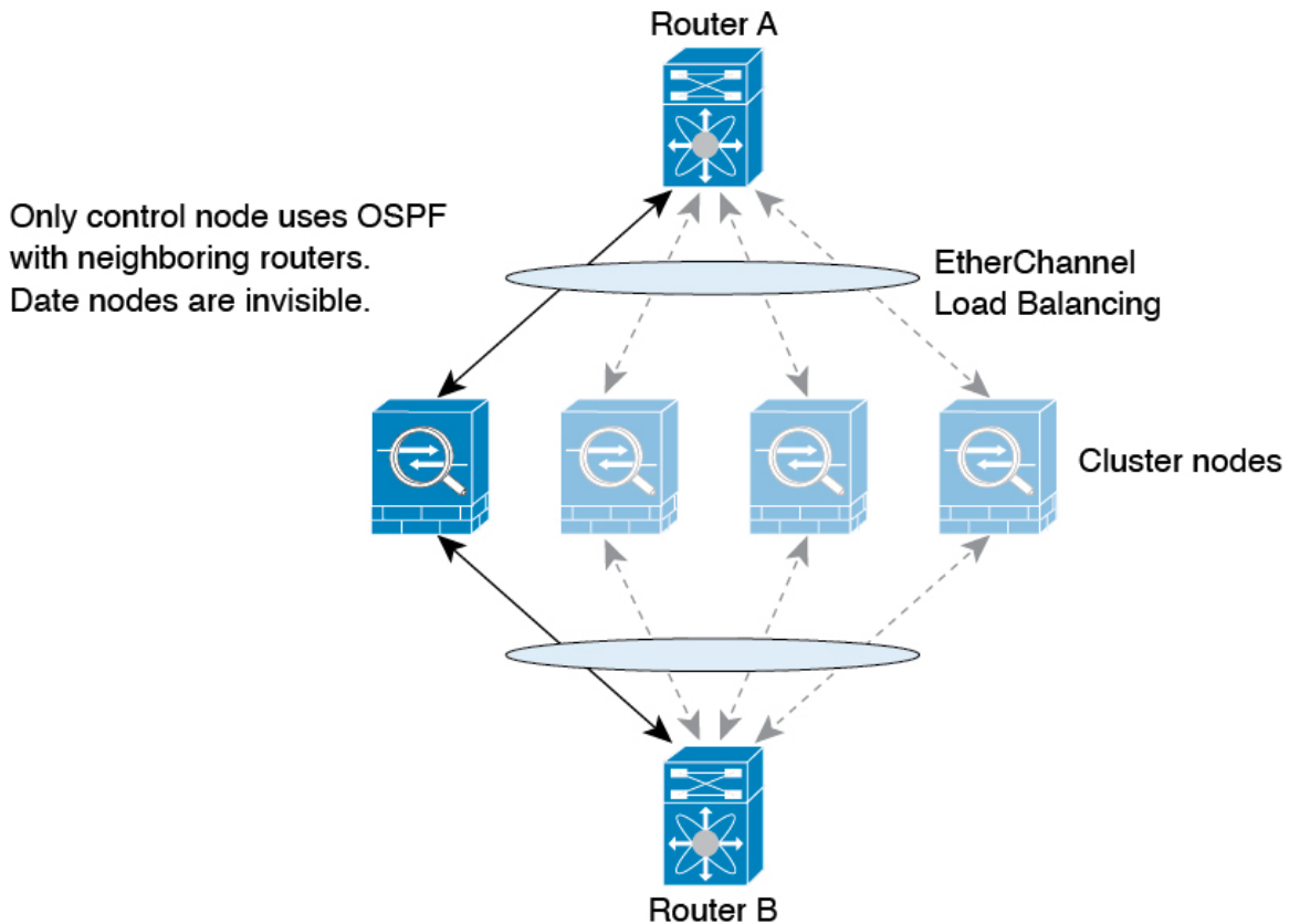
그림 29: 클러스터링의 동적 라우팅
