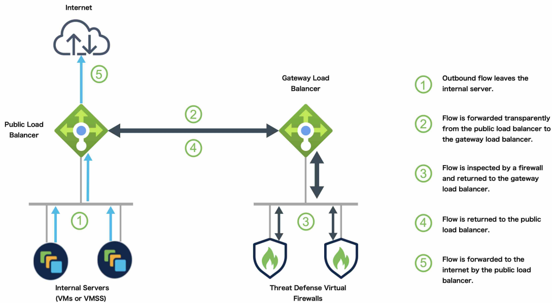
그림 2: GWLB를 사용하는 아웃바운드 트래픽 활용 사례 및 토폴로지
