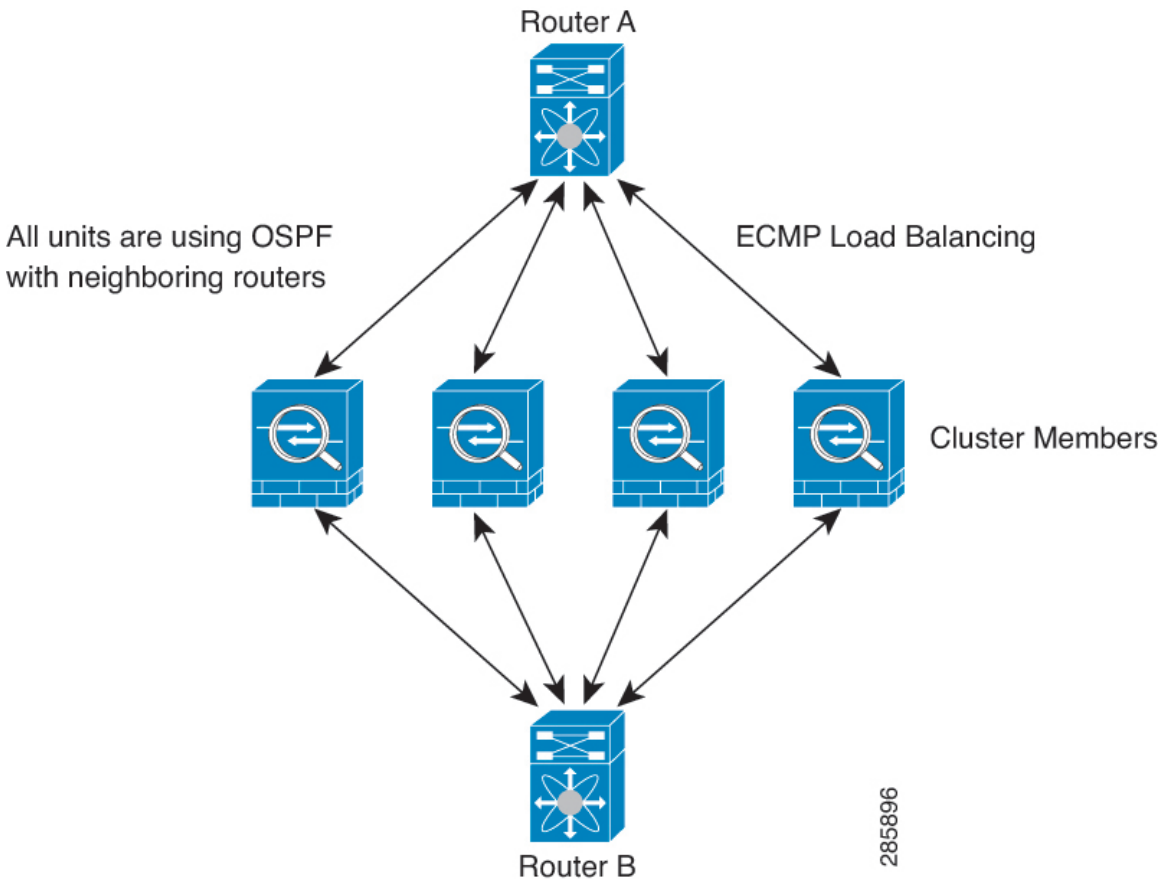
그림 20: 개별 인터페이스 모드의 동적 라우팅
