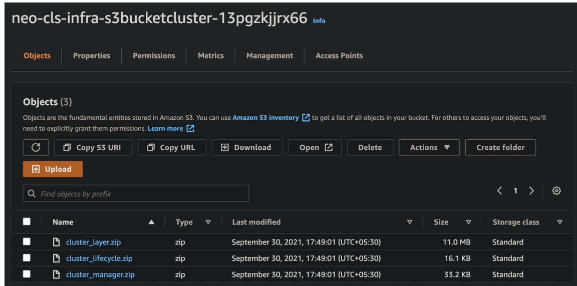
그림 3: S3 버킷
