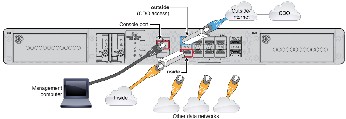
그림 63: Secure Firewall 4200 케이블 연결
