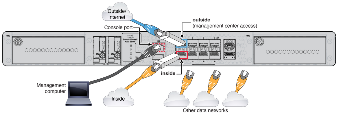
그림 34: 원격 관리 구축 케이블 연결
