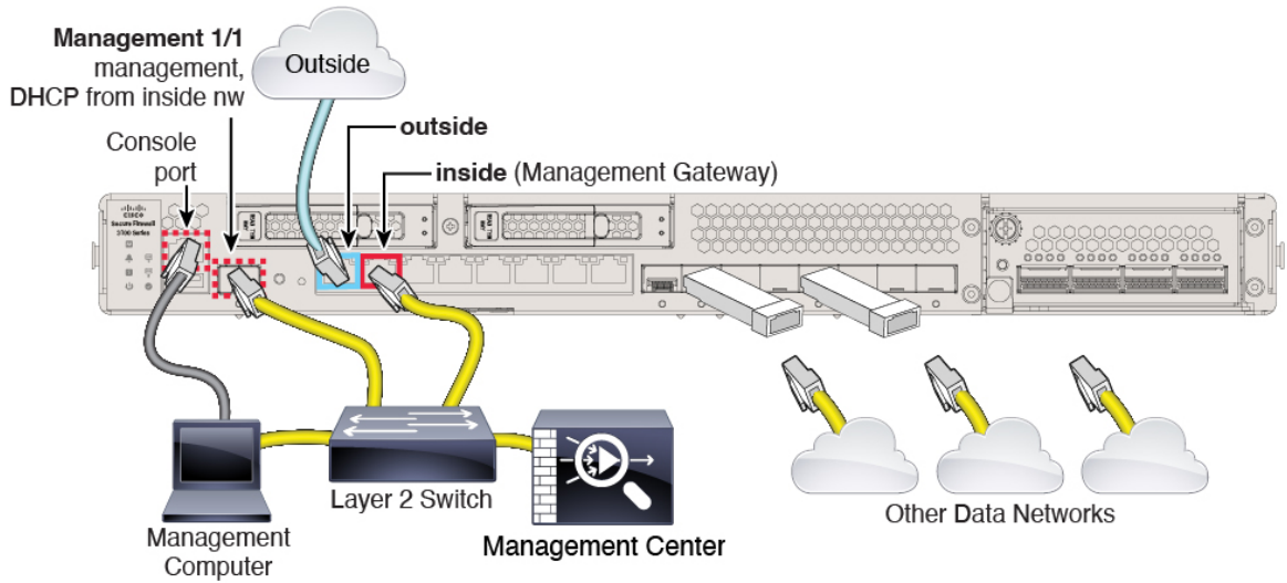
그림 5: Edge 구축 케이블 연결
