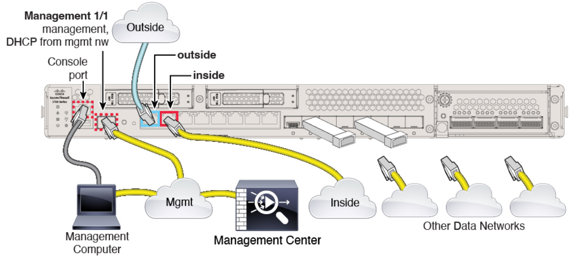
그림 4: 별도의 관리 네트워크 케이블 연결
