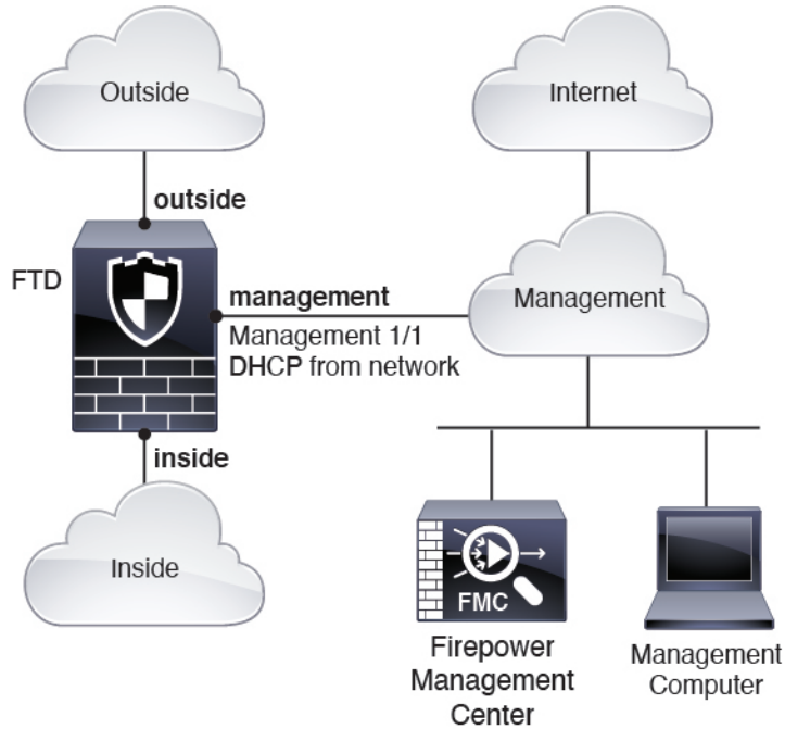
그림 2: 별도의 관리 네트워크
