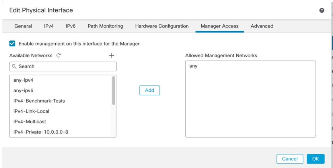
그림 4: 관리자 액세스
