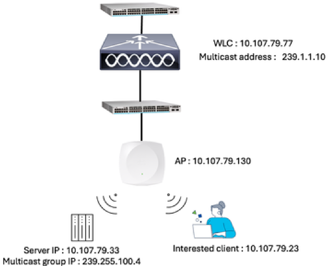
네트워크 다이어그램
