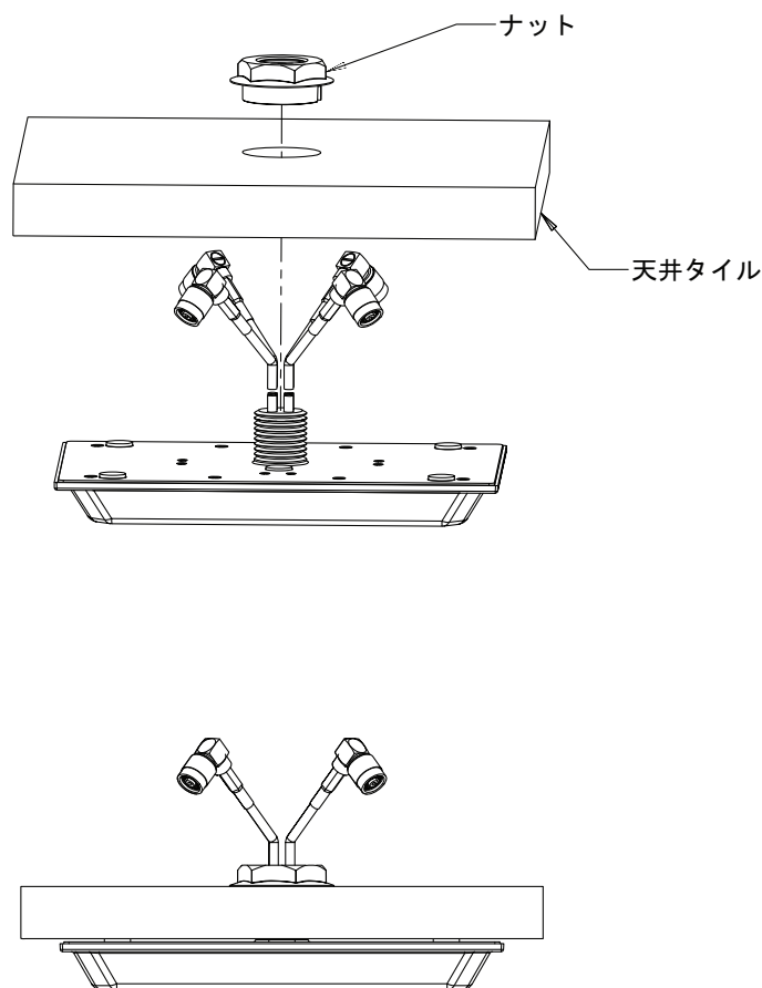
図 1 天井タイルへの取り付けの詳細
