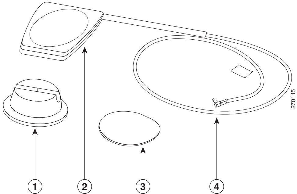
図 2 指向性アンテナ キットの内容
