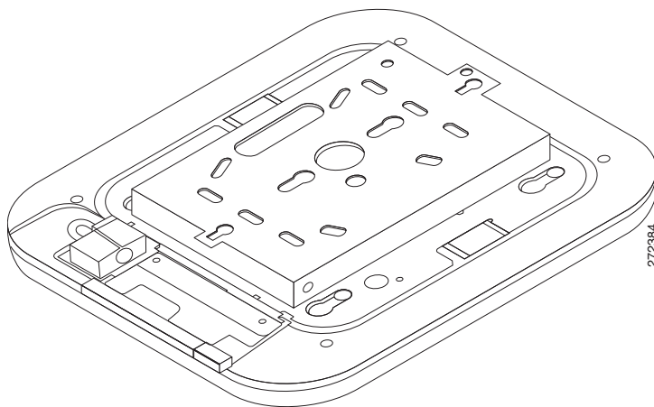
図 2 アクセス ポイントに取り付けられたユニバーサル ブラケット
