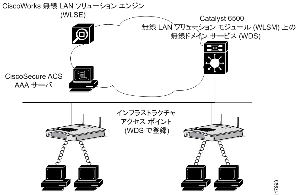
図 11-3 レイヤ 3 モビリティに必要なコンポーネント
