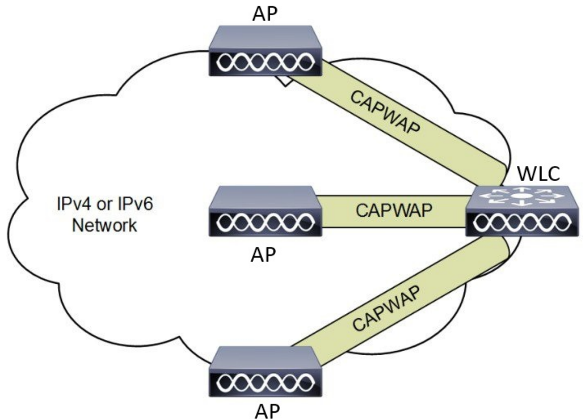
図 1: WLC に接続された CAPWAP AP
