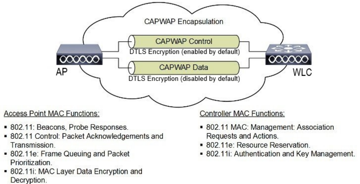
図 2: スプリット MAC アーキテクチャ
