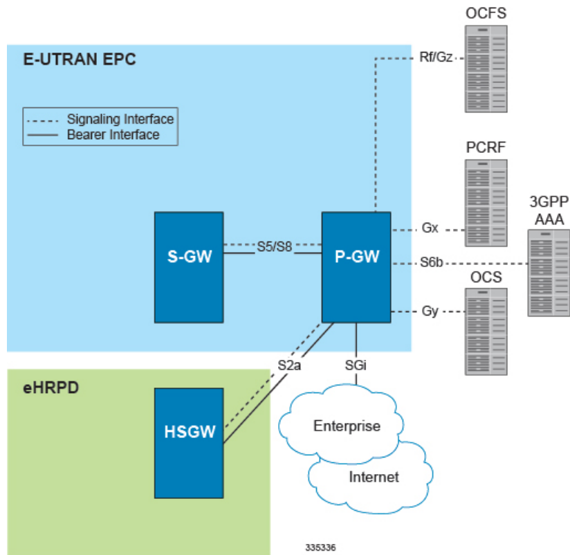
図 5: eHRPD から E-UTRAN/EPC への接続をサポートする P-GW インターフェイス
