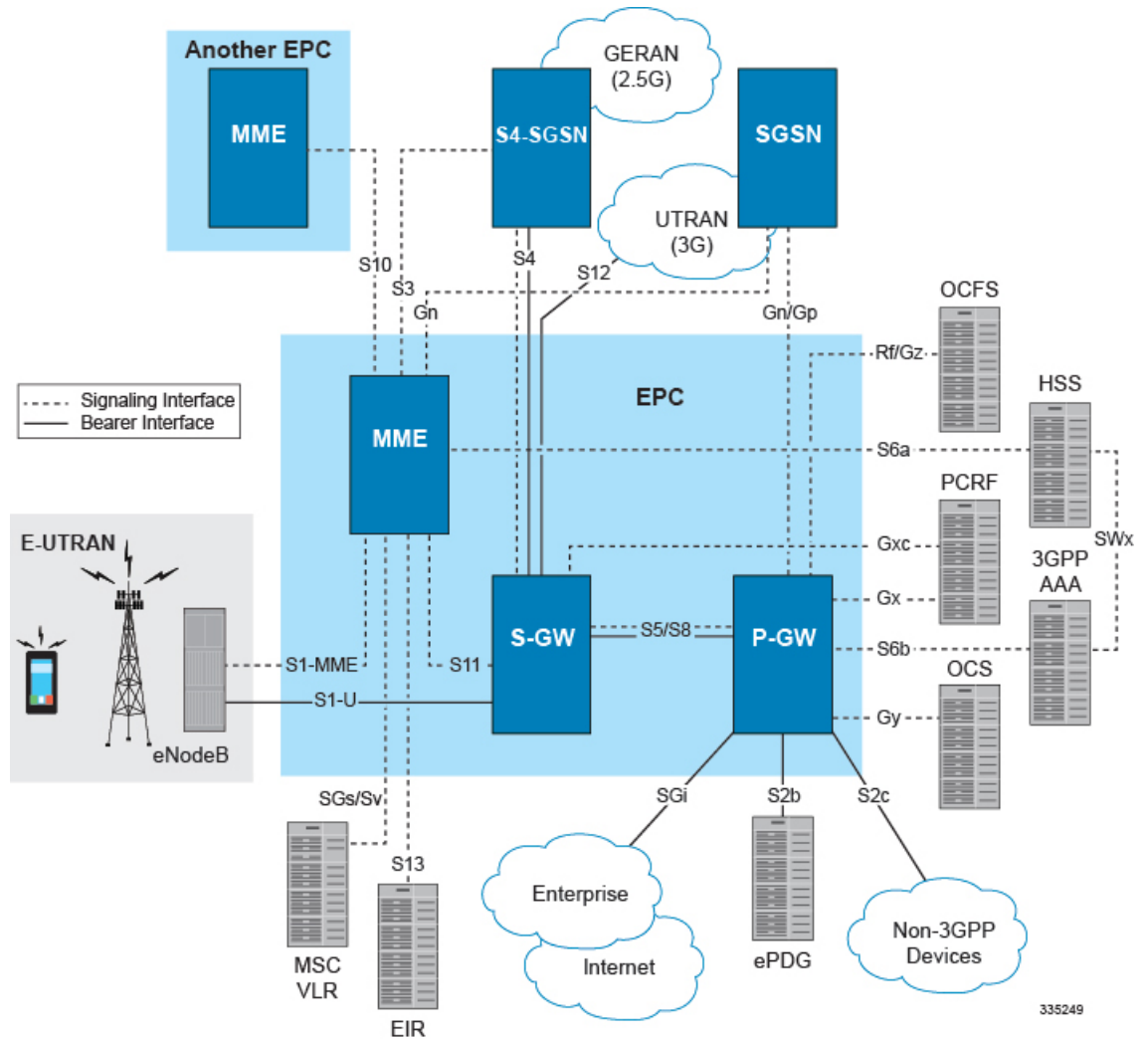
図 4: E-UTRAN/EPC ネットワークにおける P-GW
