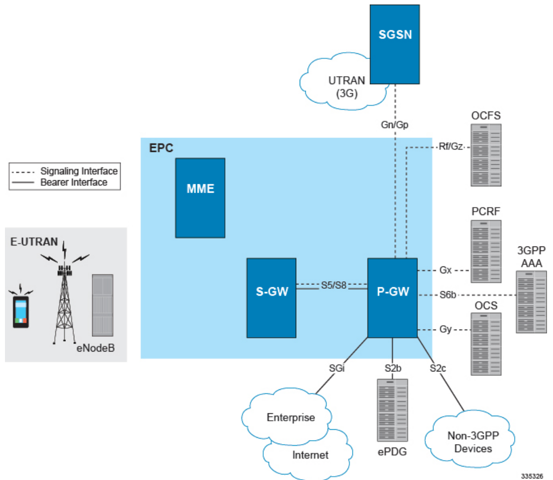
図 3: E-UTRAN/EPC ネットワークでサポートされる P-GW インターフェイス
