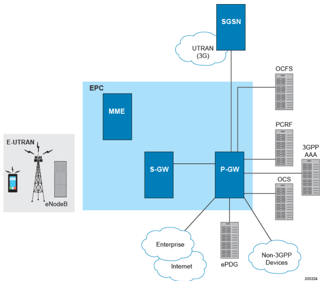
図 1: 基本的な E-UTRAN/EPC ネットワークにおける P-GW
