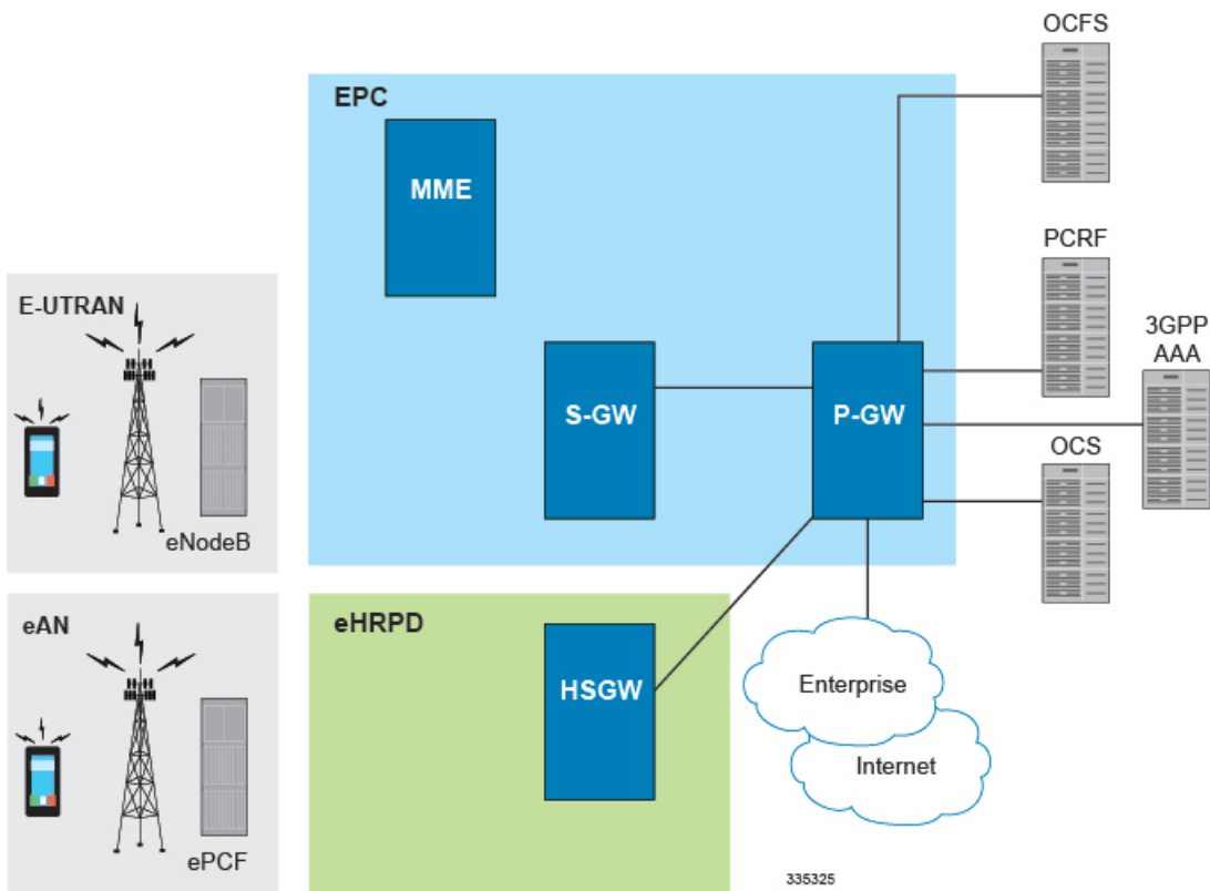
図 2: 基本的な E-UTRAN/EPC および eHRPD ネットワークにおける P-GW
