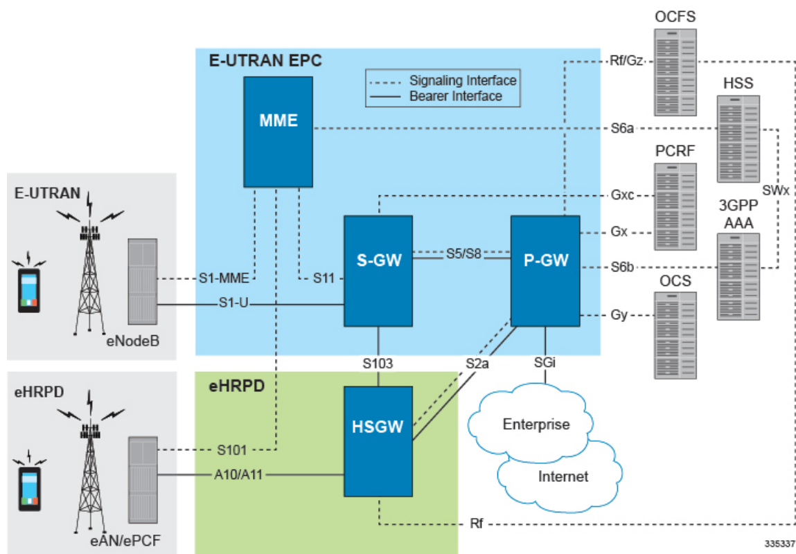
図 6: eHRPD ネットワークをサポートする E-UTRAN/EPC ネットワーク内の P-GW
