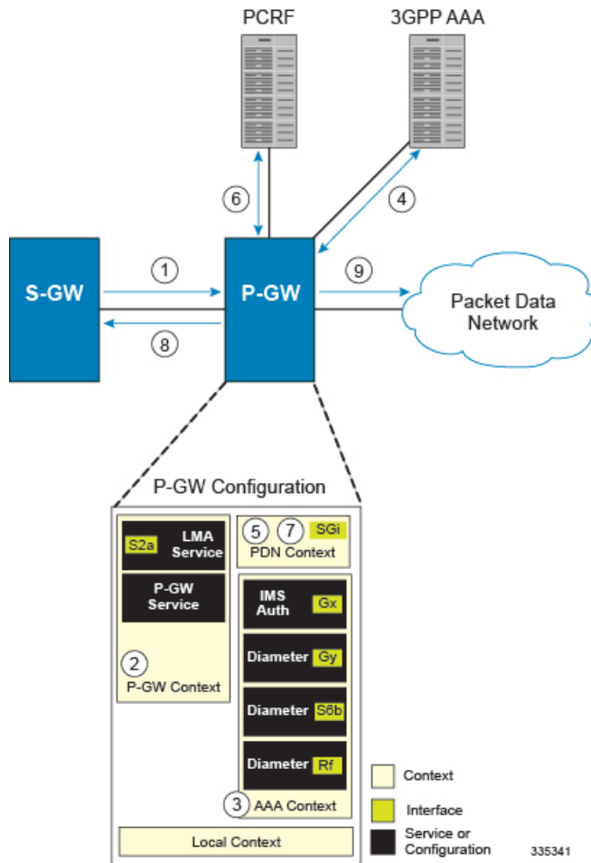
図 3: LTE ネットワークの PMIP P-GW の要素
