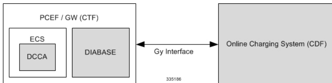
図 2: Gy アーキテクチャ
