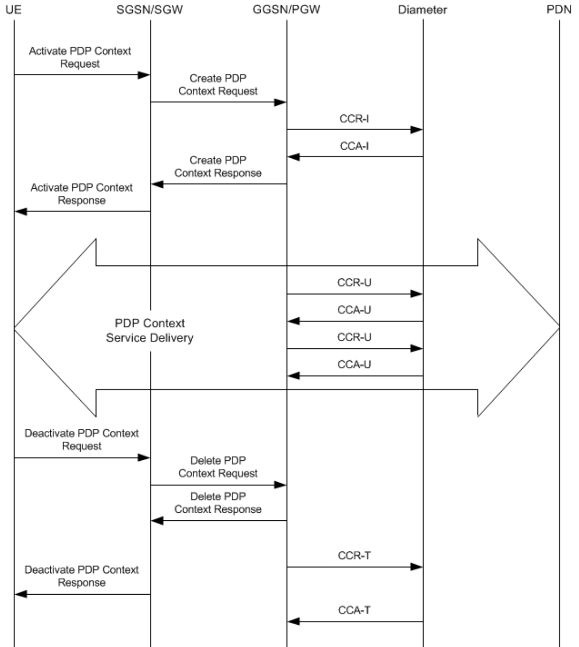
図 3: GGSN/P-GW/IPSG の単純なコール要求の Gy コールフロー
