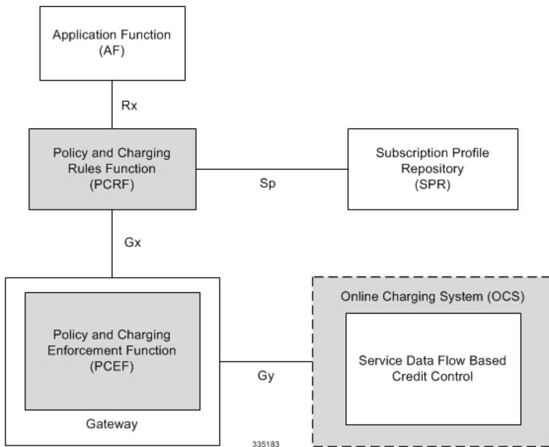
図 1: PCC 論理アーキテクチャ
