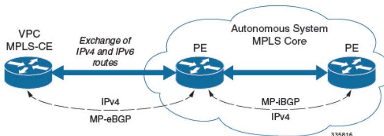
図 10: VPNv6 に対する IPv6-RD サポート
