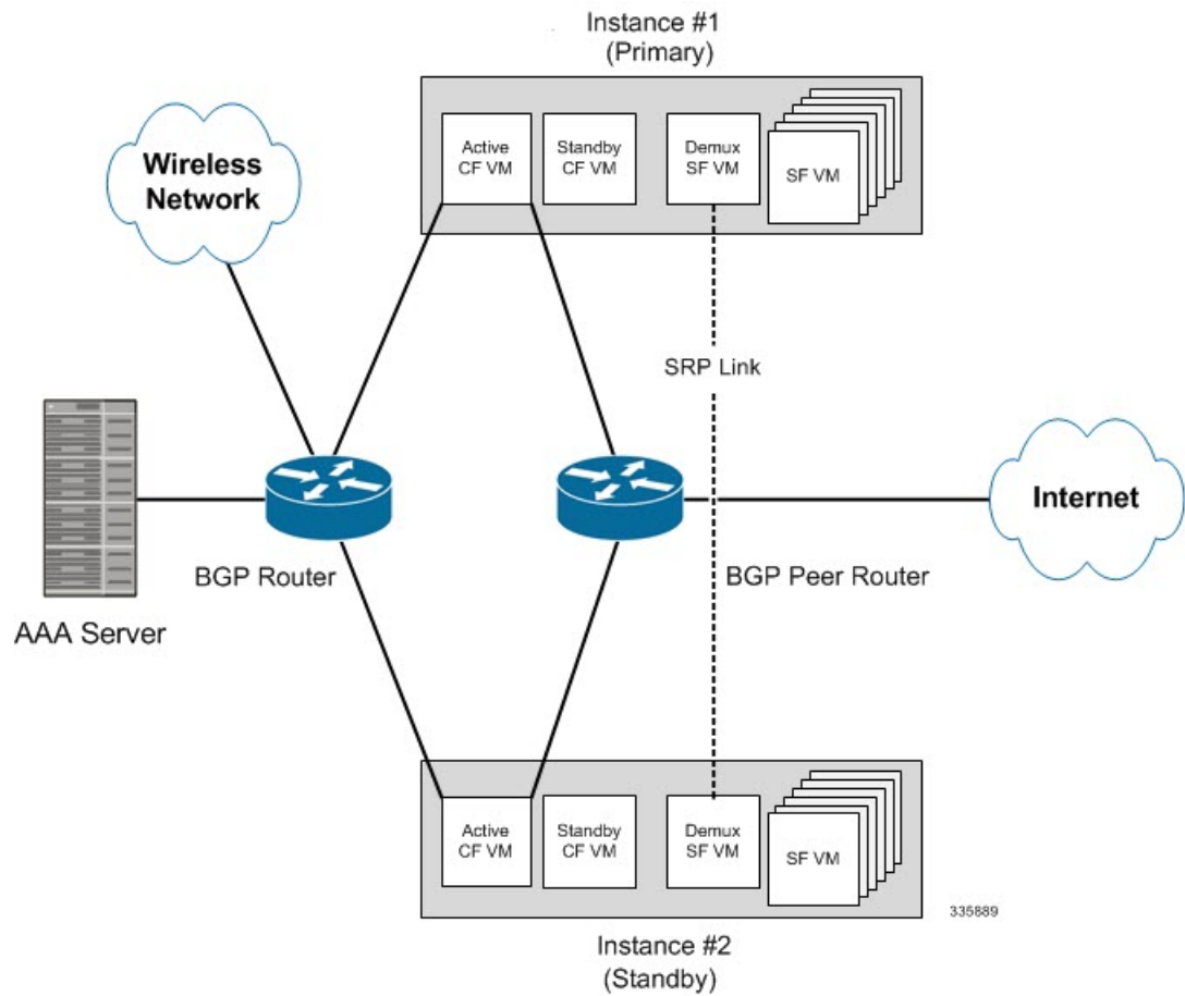
図 12: 仮想化された StarOS の ICSR のネットワーク
