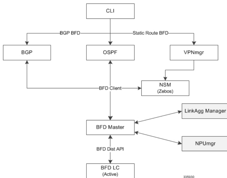
図 6: BFD の連携動作
