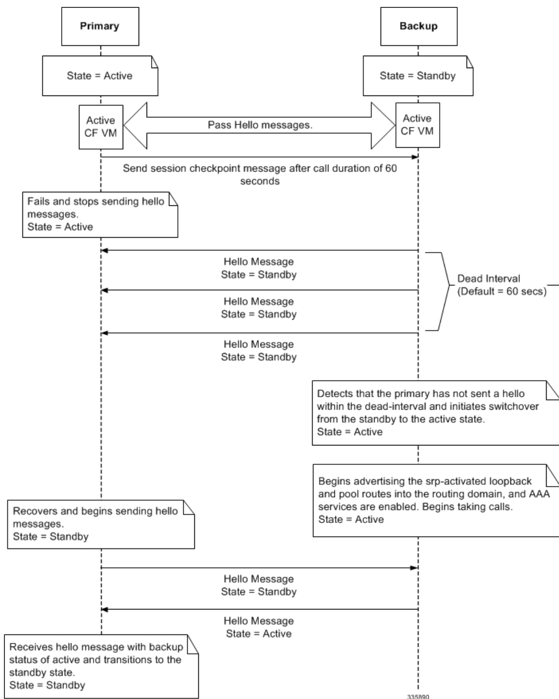
図 13: ICSR プロセスフロー (プライマリ障害)
