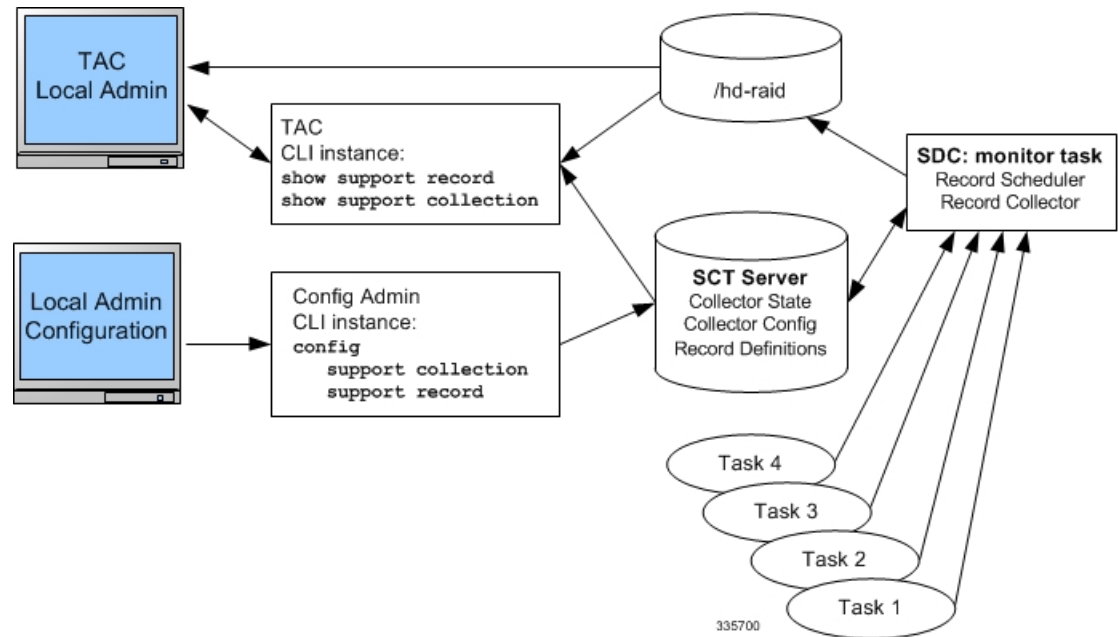
図 20: SDC のタスクとプロセス
