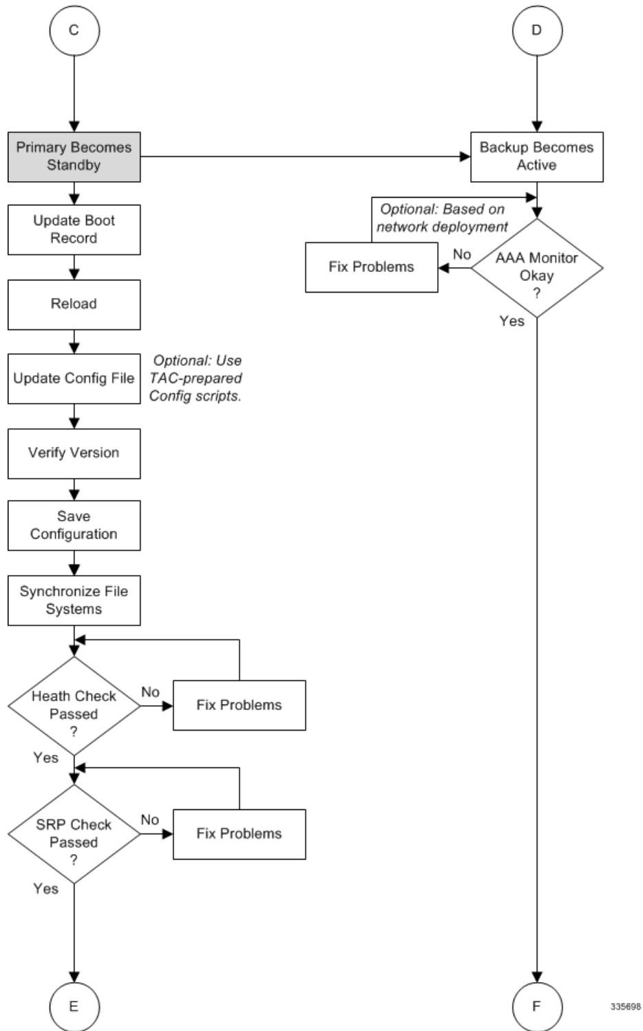
図 18: ICSR ソフトウェアアップグレード : パート3
