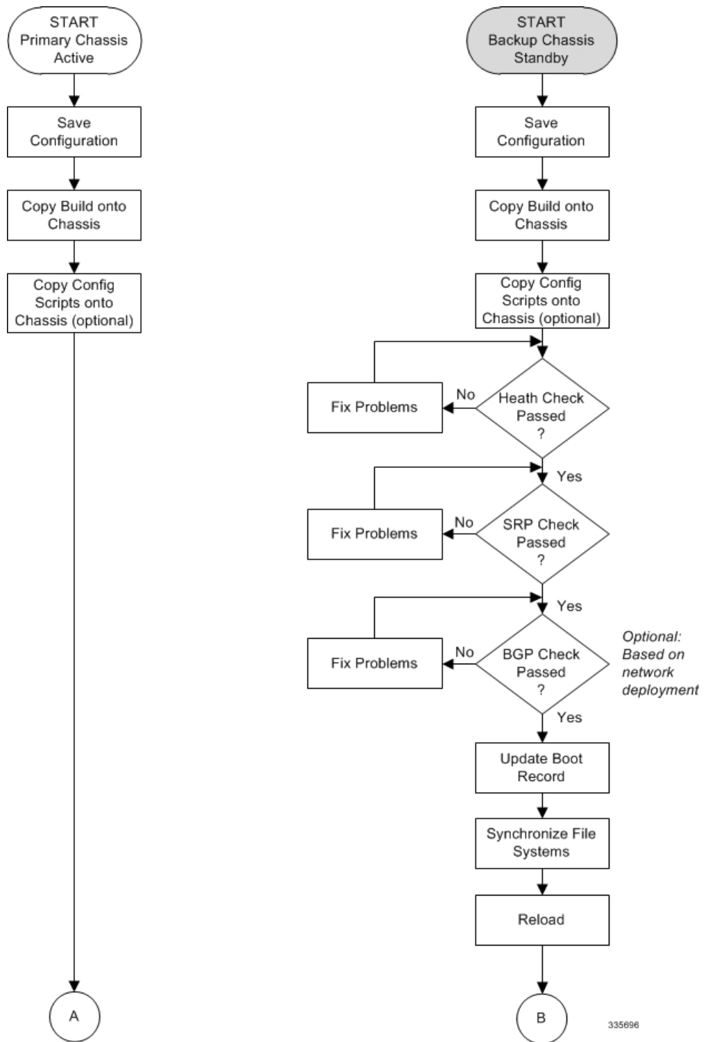
図 16: ICSR ソフトウェアアップグレード : パート 1
