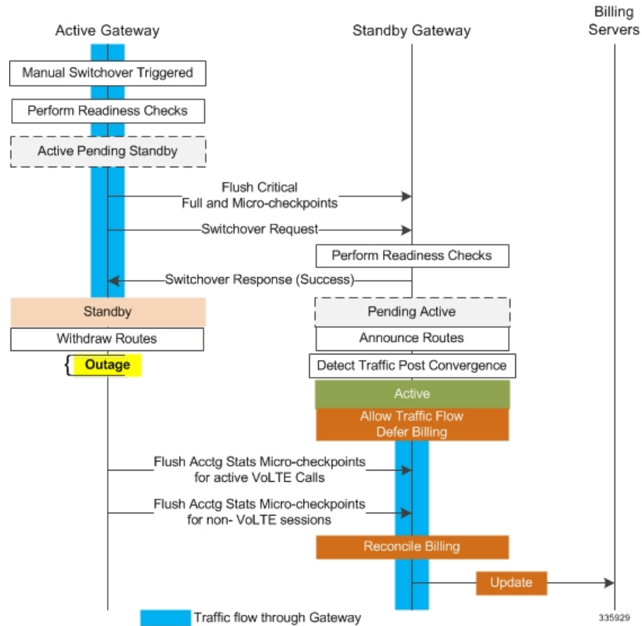
図 15: コールフロー : 非 VoLTE データ停止の削減
