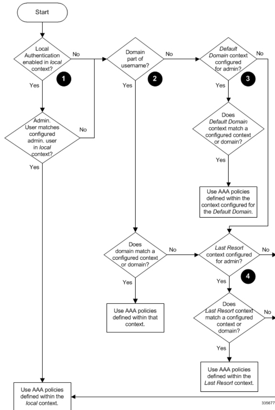
図 4: コンテキストレベルの管理ユーザの AAA コンテキスト
