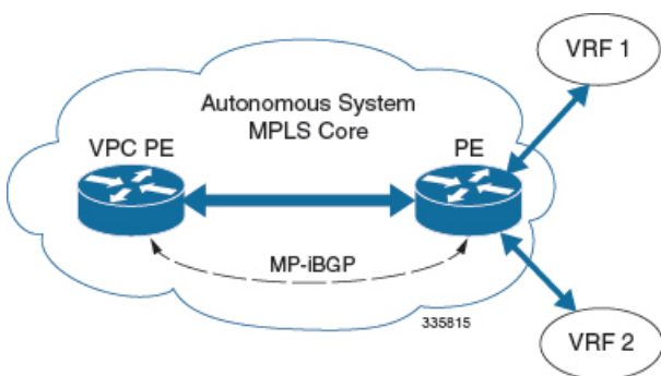
図 9: 設定例
