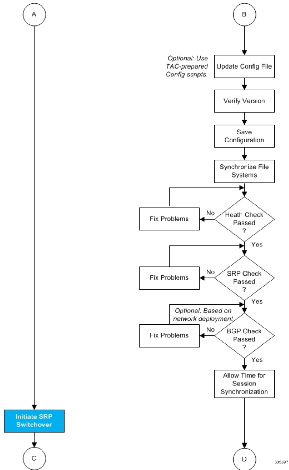
図 17: ICSR ソフトウェアアップグレード : パート2
