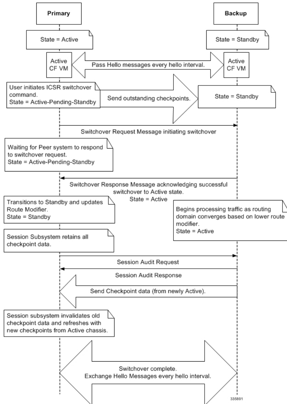
図 14: ICSR プロセスフロー (手動スイッチオーバー)
