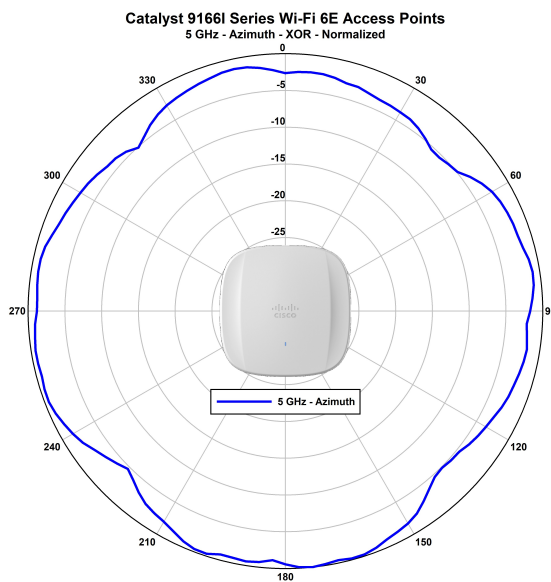
図 9: CW9166I - XOR 正規化放射パターン (5 GHz 水平)
