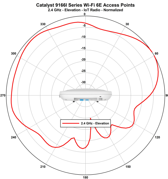
図 18: CW9166I - IoT (BLE) アンテナ正規化放射パターン (2.4 GHz 垂直)
