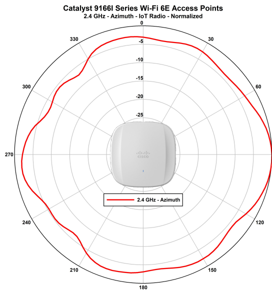
図 17: CW9166I - IoT (BLE) アンテナ正規化放射パターン (2.4 GHz 水平)
