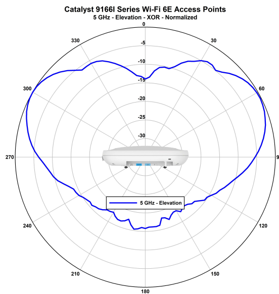
図 10: CW9166I - XOR 正規化放射パターン (5 GHz 垂直)
