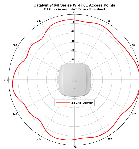
図 15: CW9164I - IoT (BLE) アンテナ正規化放射パターン (2.4 GHz 水平)
