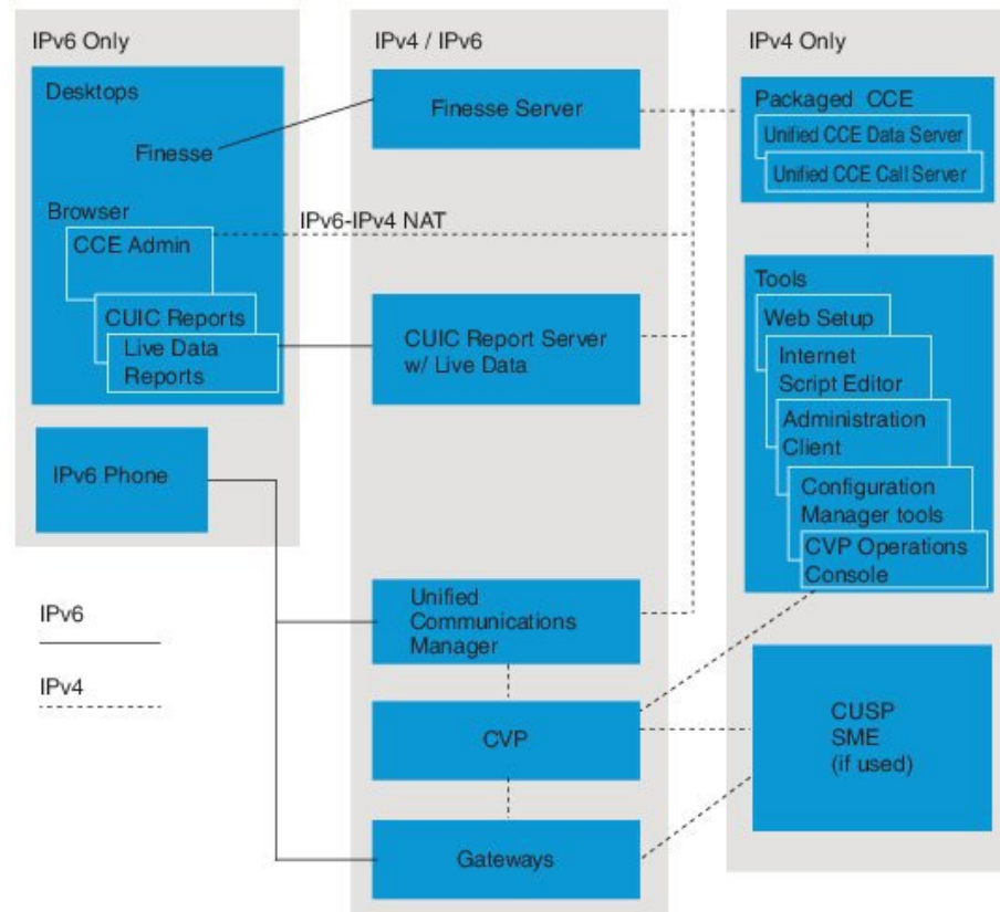
図 2: IPv6 エージェントのみを配置する Packaged CCE の展開
