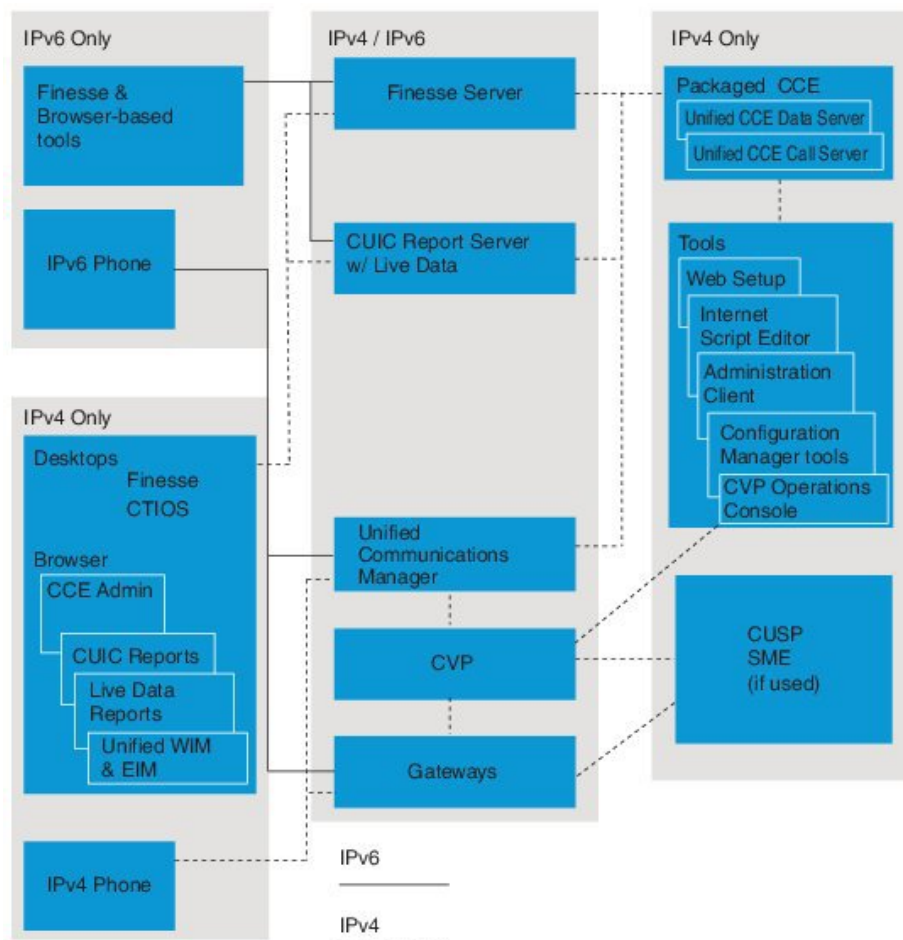
図 3: IPv4 および IPv6 の両方を使用するエージェントを配置する Packaged CCE の展開
