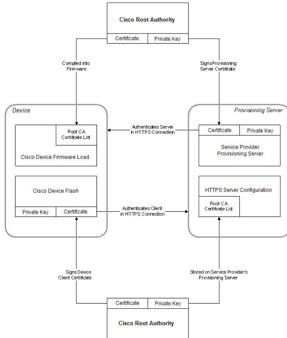
図 8: 認証局のフロー
