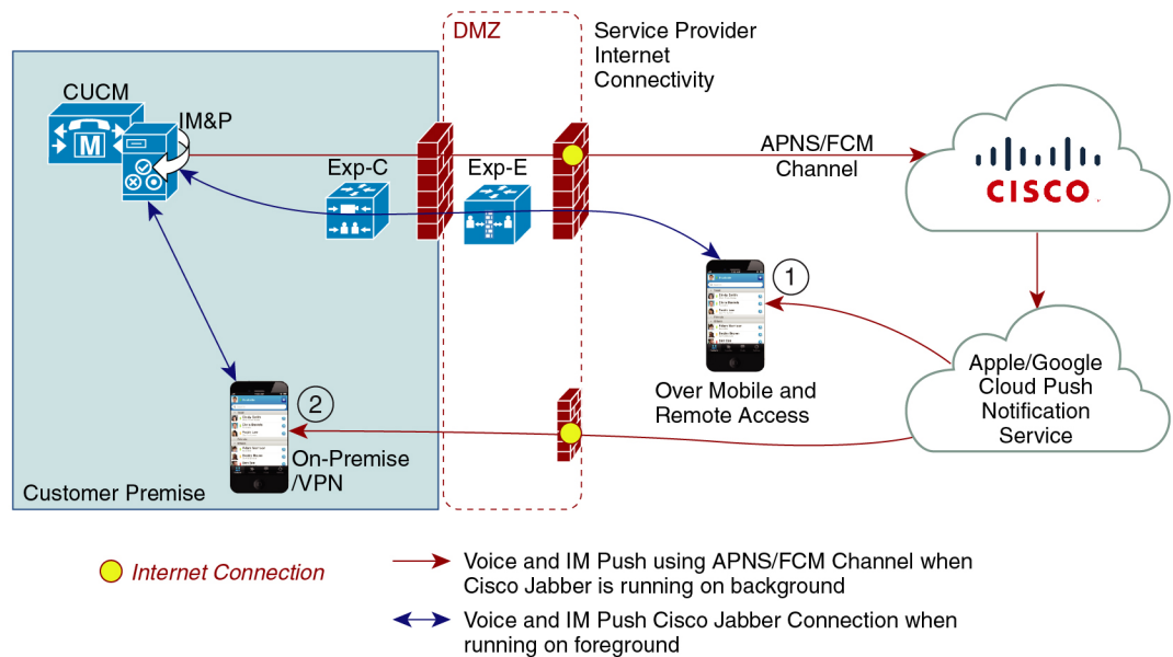
図 1: プッシュ通知のアーキテクチャ
