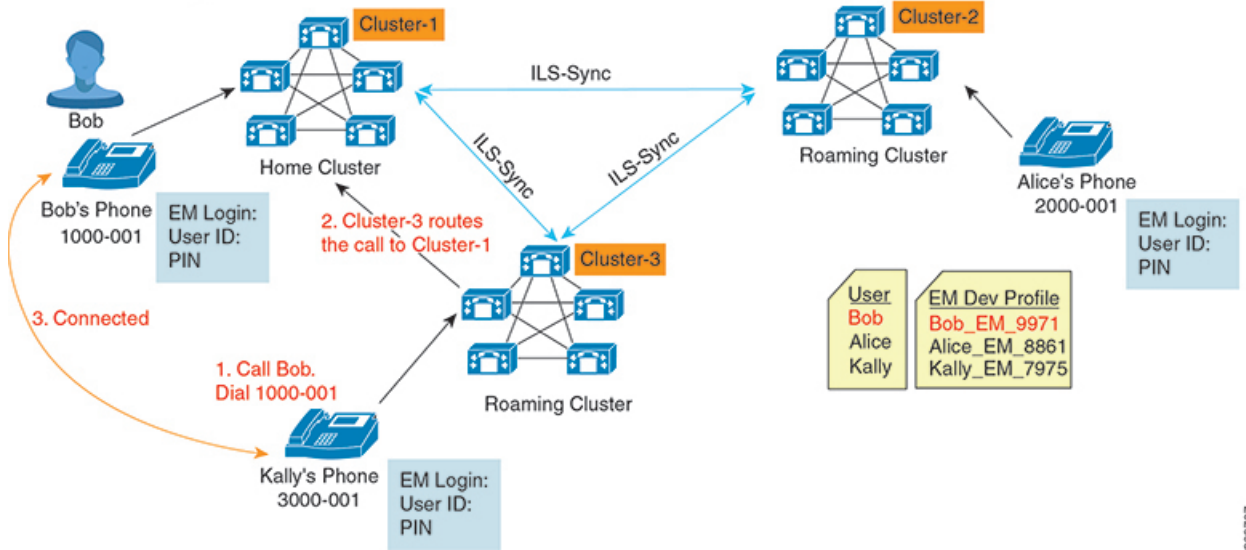
図 2: ユーザがホーム クラスタにいる場合のコール フロー
