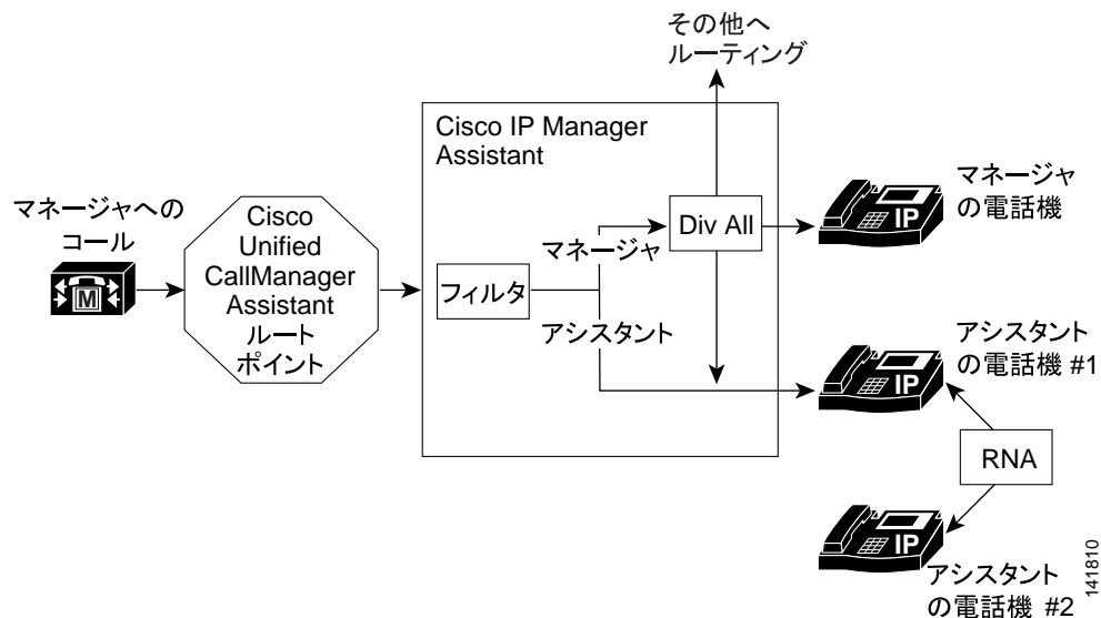
図 9-2 プロキシ回線サポート用の Cisco Unified Communications Manager Assistant のルーティング ロジック
