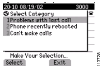
図 29-5 QRT Phone Interface : オンフック、対話モードの表示
