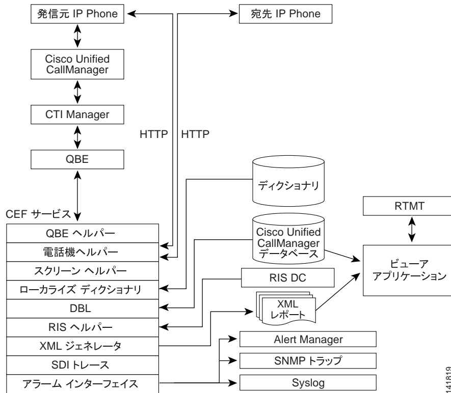
図 29-1 Cisco Extended Functions サービスのアーキテクチャの使用
