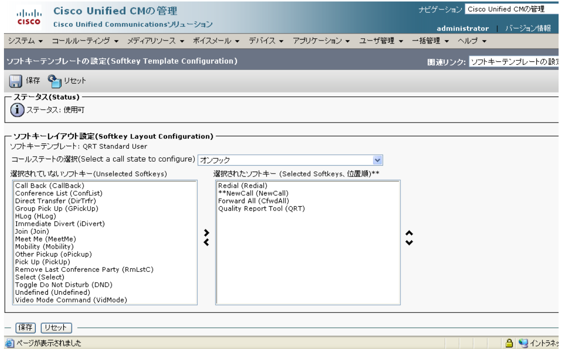
図 29-12 QRT [ソフトキーレイアウト設定 (Softkey Layout Configuration)] ウィンドウ
