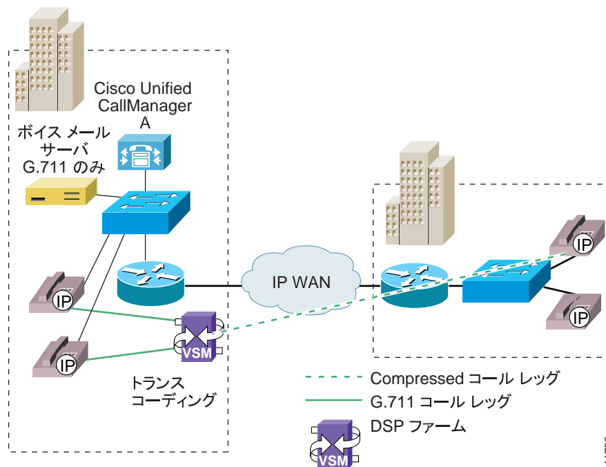
図 26-1 中央集中型 MTP トランスコーディング サービスおよび会議サービスを使用する複数サイト WAN
