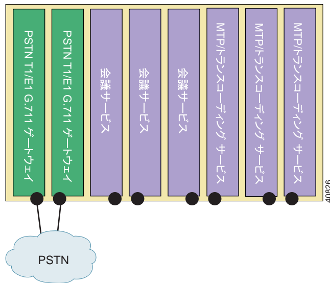
図 26-2 Cisco Catalyst 6000 音声ゲートウェイ モジュール
