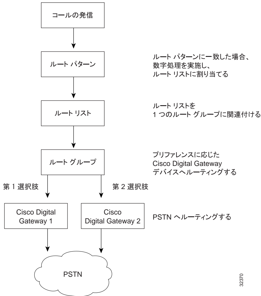
図 15-2 Cisco Digital Gateway 用のルートプランの要約図
