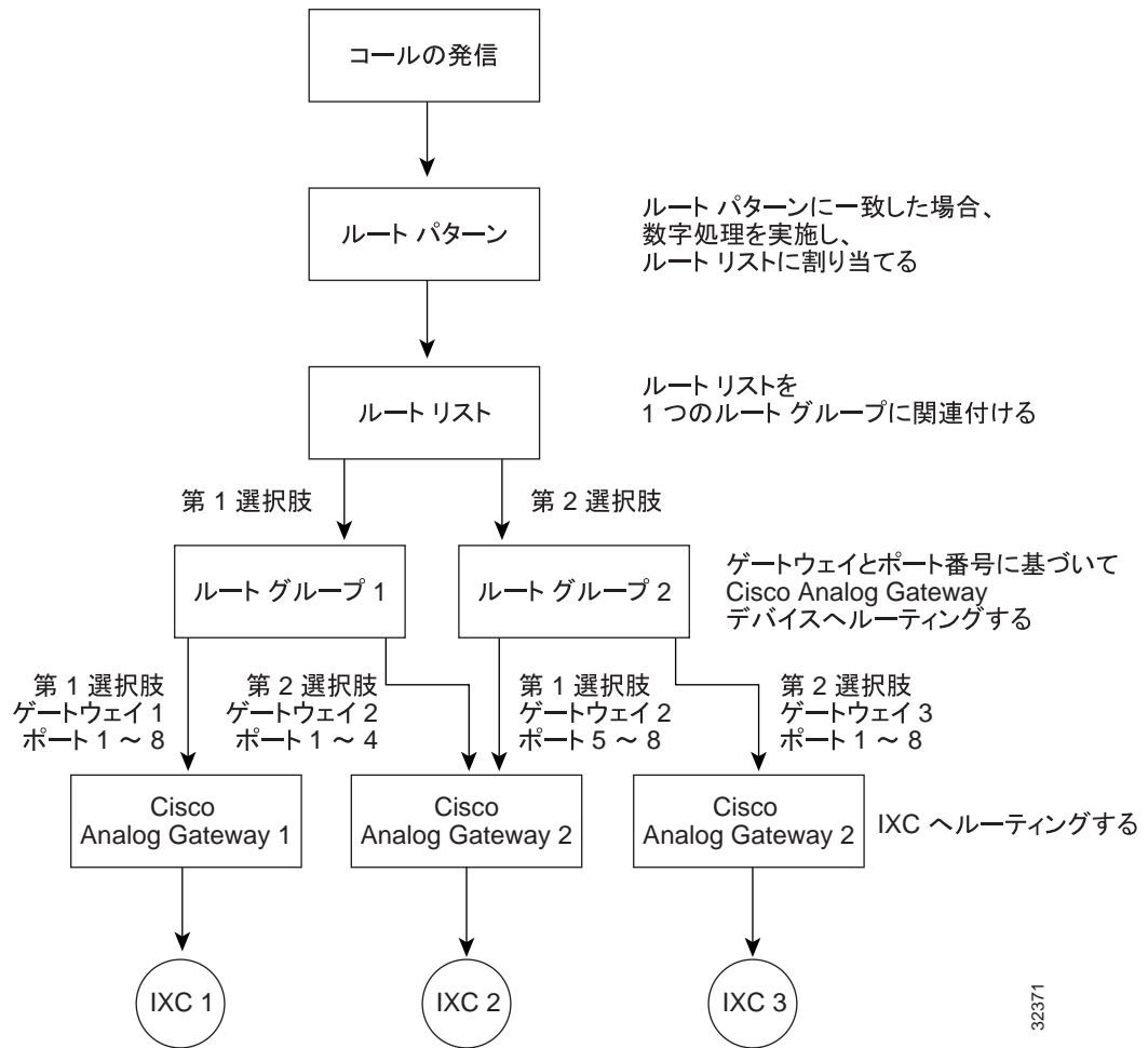
図 15-3 Cisco Analog Access Gateway 用のルートプランの要約図
