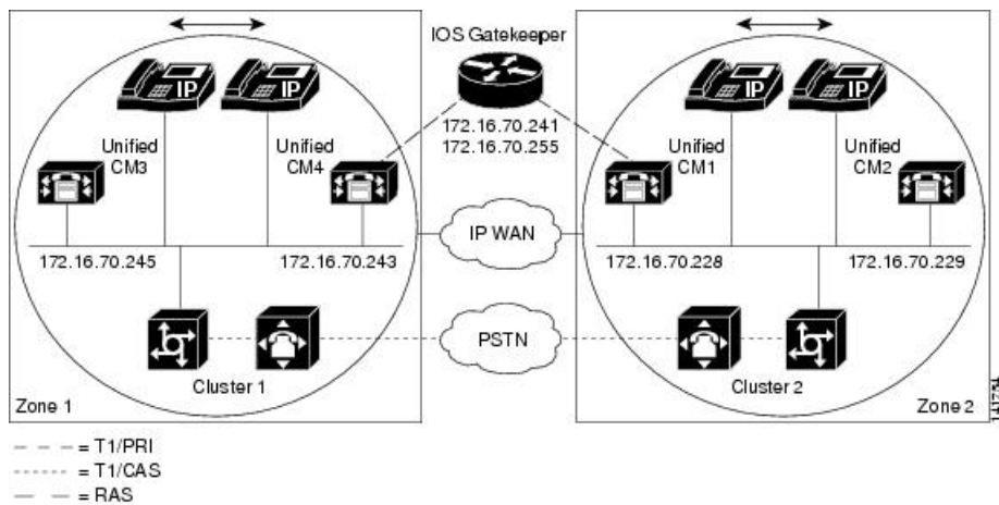
図 1：クラスタ内の Cisco Unified IP Phone と Cisco Unified IP Phone 間のコールのサンプルトポロジ
