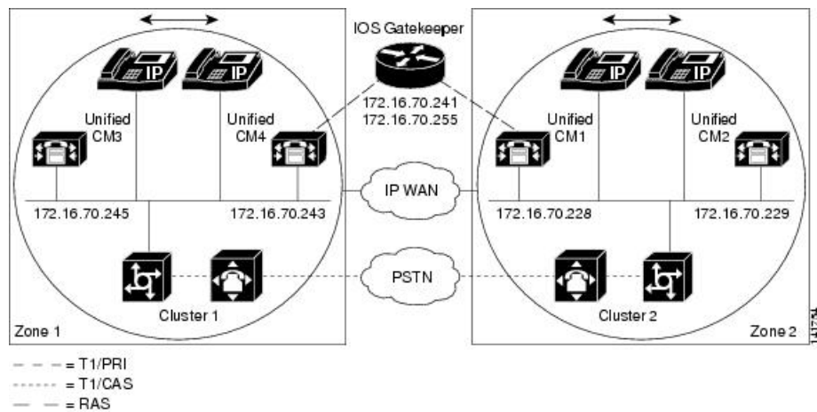
図 2：クラスタ内の Cisco Unified IP Phone と Cisco Unified IP Phone 間のコールのサンプルトポロジ
