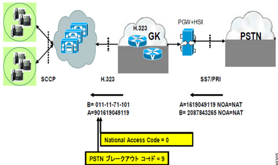
図 1-5 PSTN から IP 電話への着信コール
