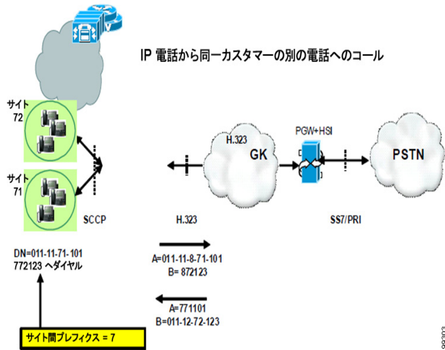
図 1-3 H.323 インターフェイスにおける、サイト間コールと関連付けられている 2 つのコール レッグ に対する番号付け
