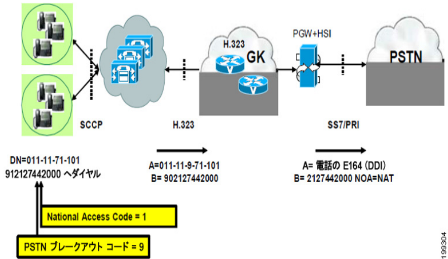
図 1-4 Unified CM と Cisco PGW 間のインターフェイスにおける、アメリカでのナショナル PSTN コールに対する番号付け
