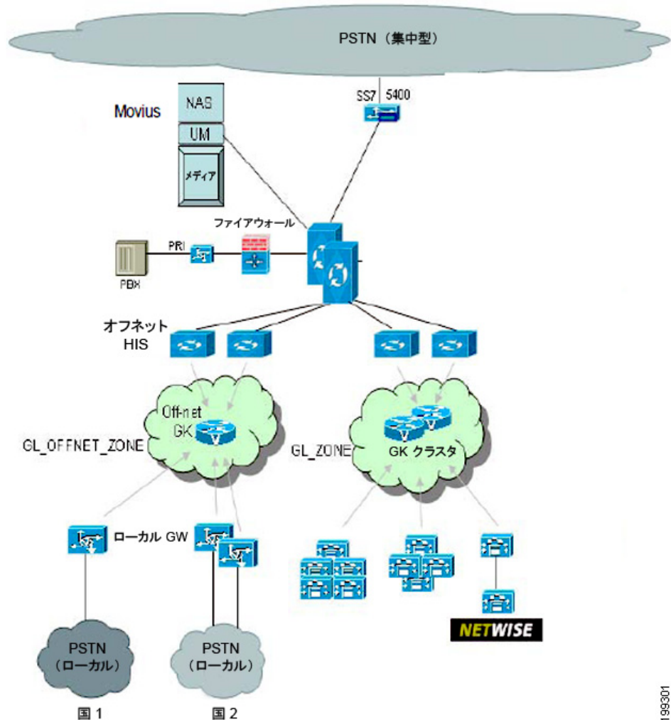
図 1-1 ホステッド UCS システム
