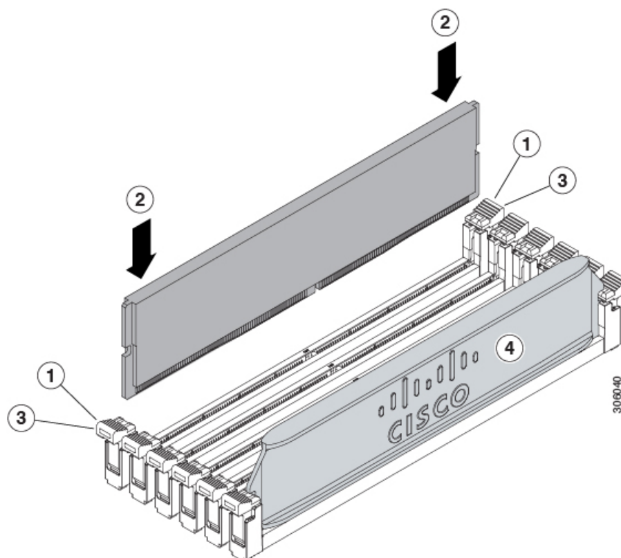
図 9: メモリの取り付け
