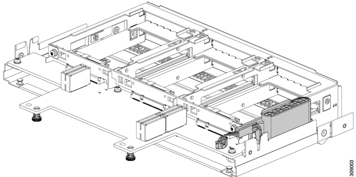
図 7: SuperCap モジュールの位置
