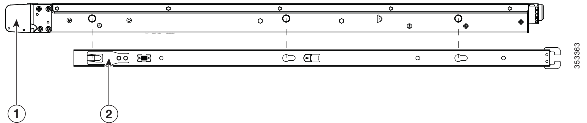
図 2-1 サーバの側面への内側レールの装着
