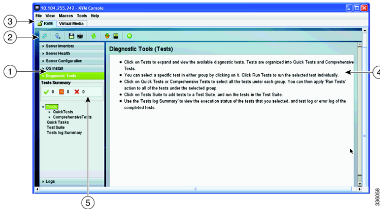
図 3-1 UCS-SCU GUI
