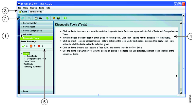
図 3-1 UCS-SCU GUI
