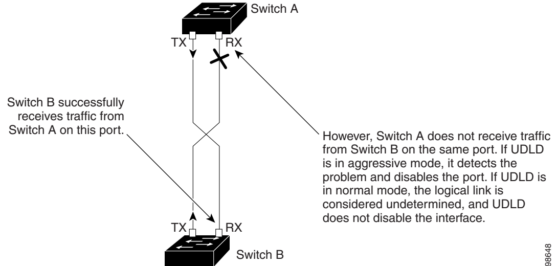
図 71 UDLD による単一方向リンクの検出
