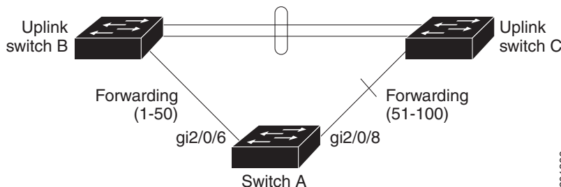
図 58 VLAN FlexLink ロード バランシングの設定例
