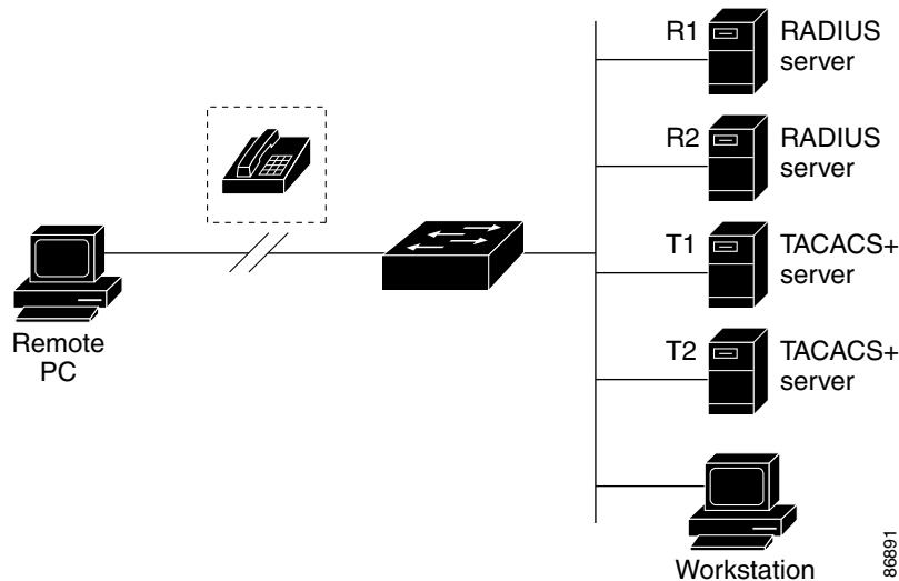
図 17 RADIUS サービスから TACACS+ サービスへの移行
