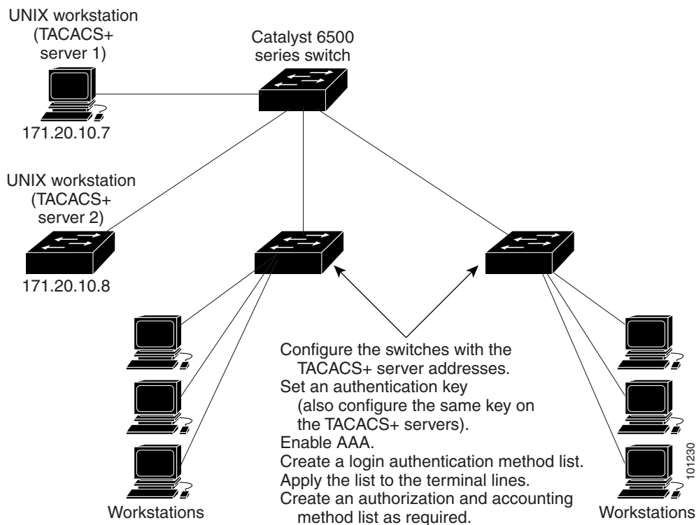
図 16 一般的な TACACS+ ネットワーク構成
