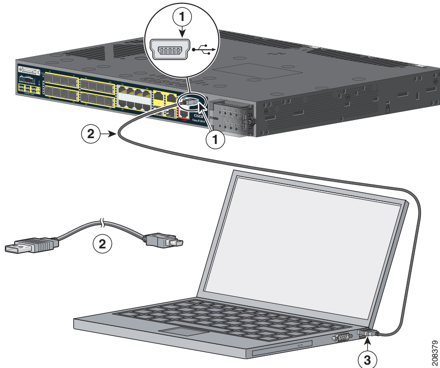
図 24 USB コンソール ケーブルの接続
