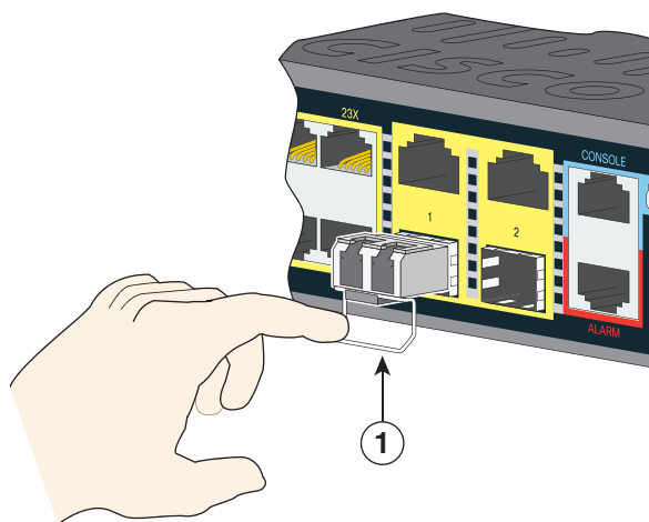
図 13 ベールクラスプ ラッチ SFP モジュールの取り外し
