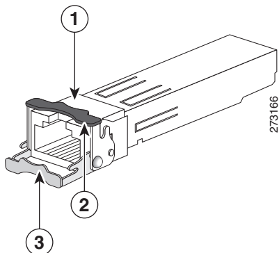
図 12 1000BASE-T SFP トランシーバ
