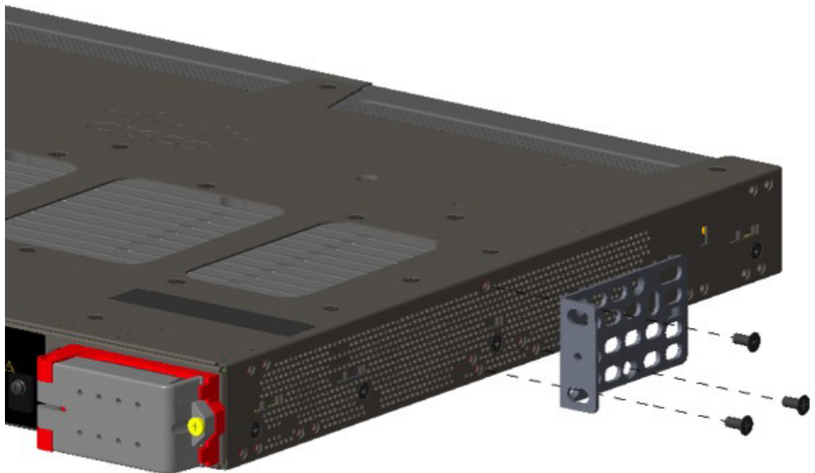
図 2 19 インチ ラック用ブラケットの取り付け(中間取り付け)
