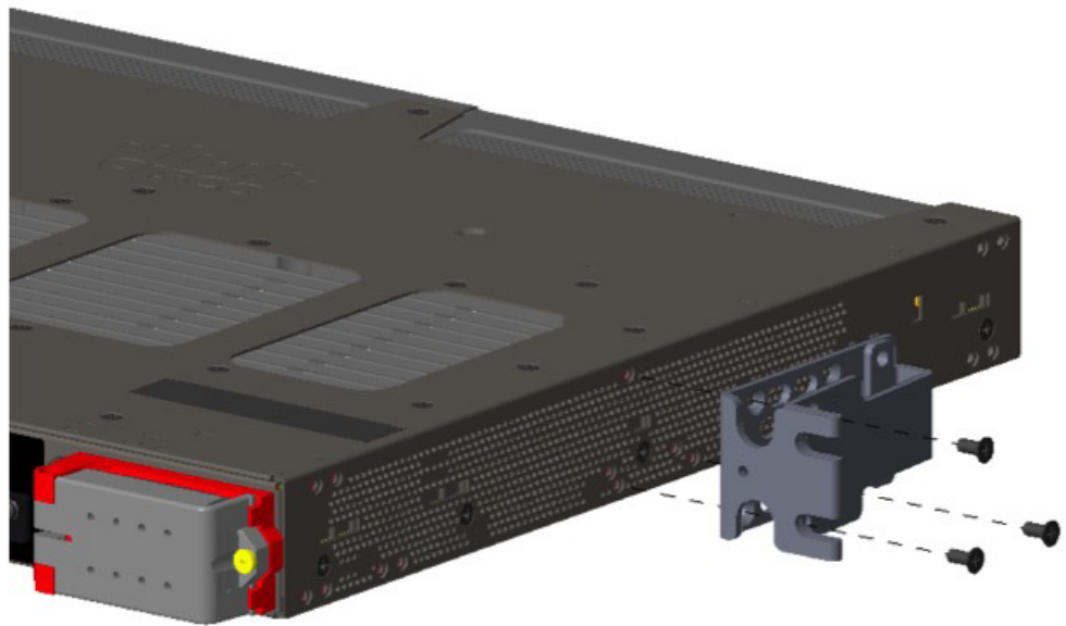
図 6 23 インチ ブラケットの取り付け
