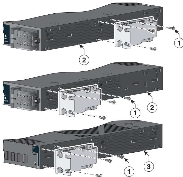
図 7 ETSI ラックのブラケット (RM-RGD-ETSI=) の取り付け
