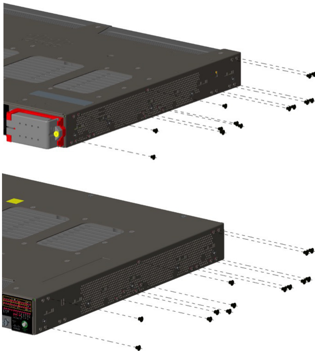
図 5 取り付け位置ごとのゴム製プラグの挿入位置
