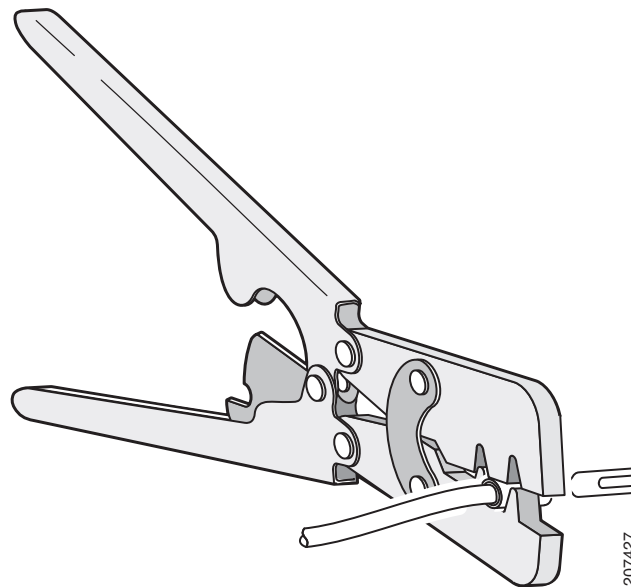
図 18 スペード端子ラグの圧着
