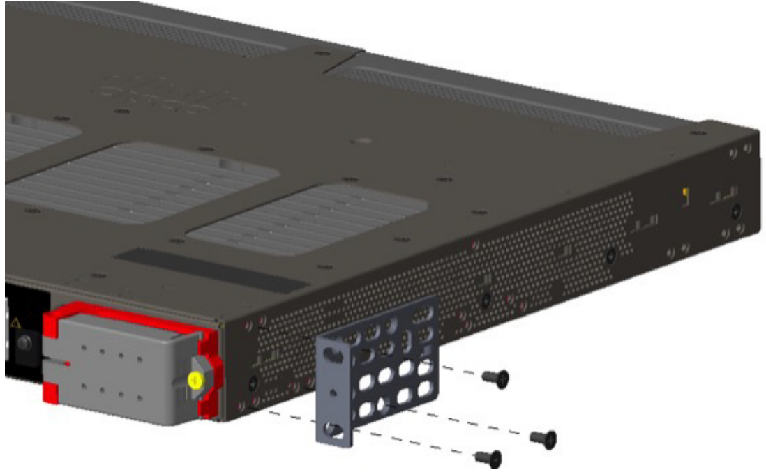
図 2 19 インチ ラック用ブラケットの取り付け(中間取り付け)
