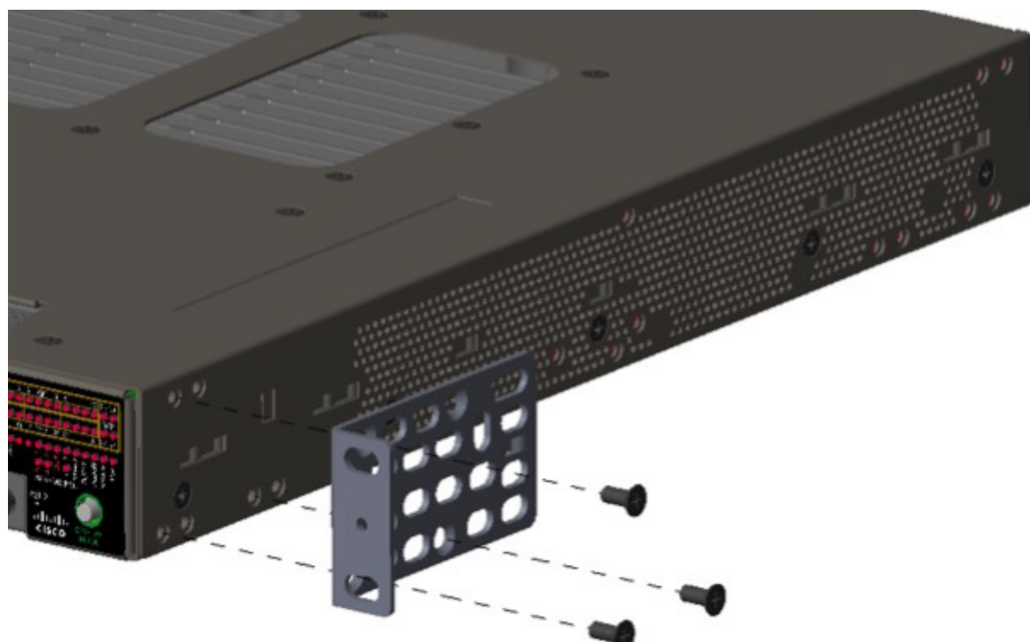
図 3 19 インチ ラック用ブラケットの取り付け(背面取り付け)
