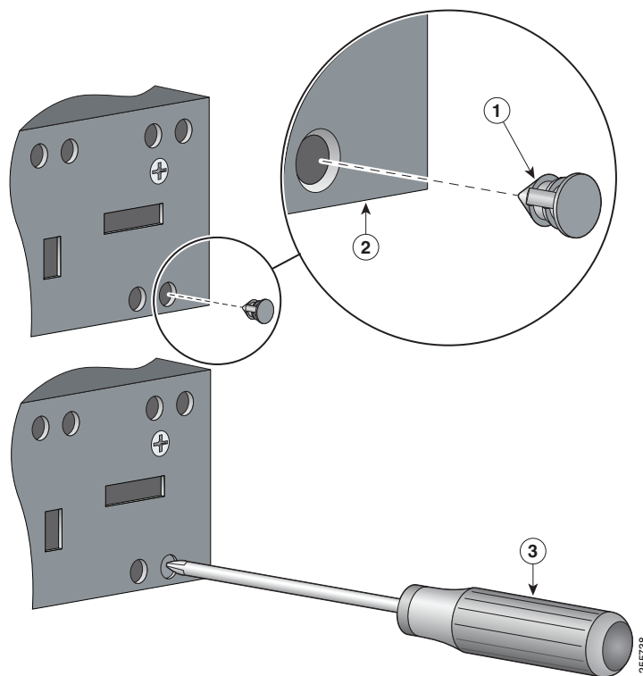
図 4 ゴム製プラグの挿入
