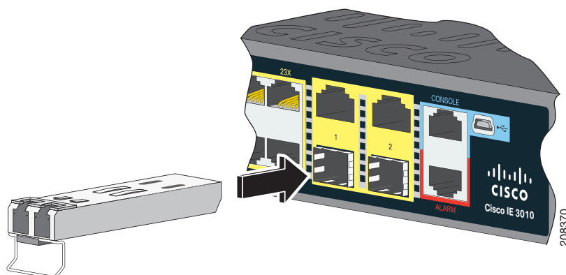
図 11 SFP モジュールの装着
