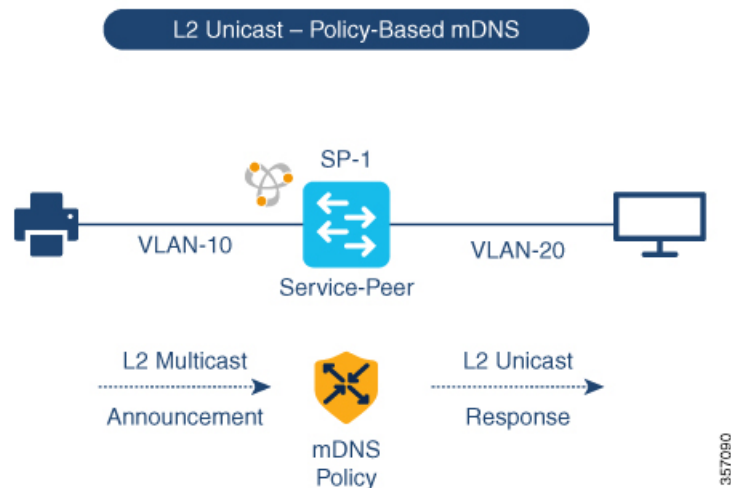
図 16: 複数 VLAN ユニキャストモードの Bonjour ネットワーク
