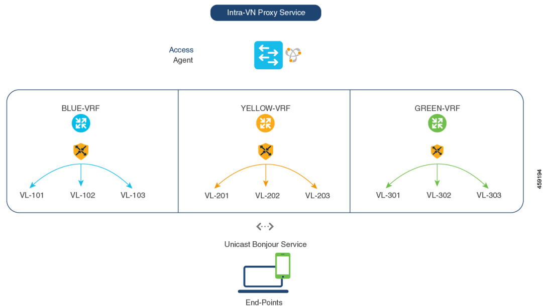
図 24: VN 間サービスプロキシ
